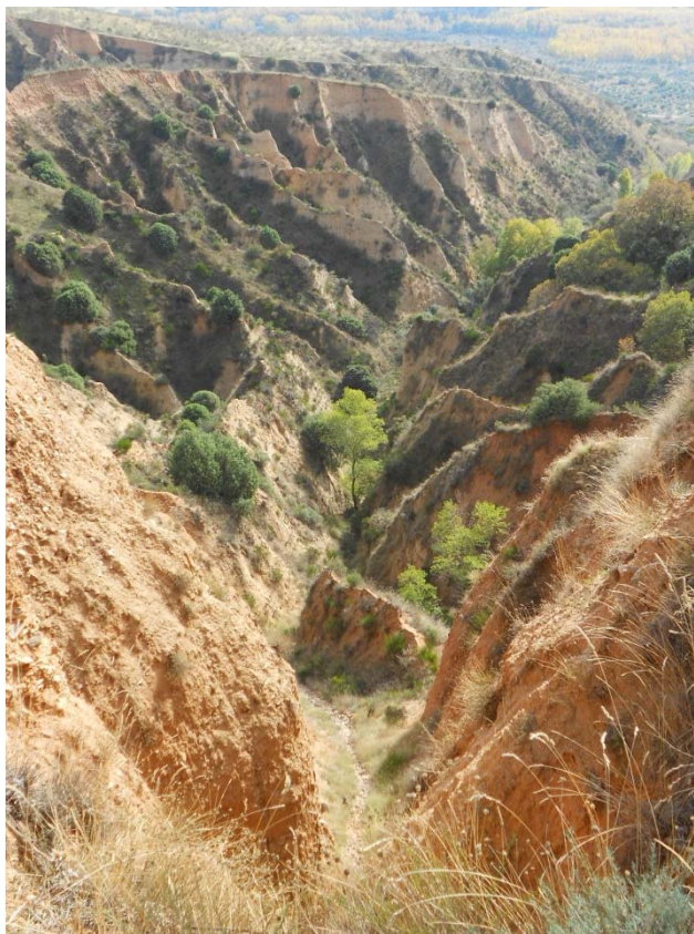
Figura o Foto 23: Cárcava del Cerro Negro desde la zona Norte.
