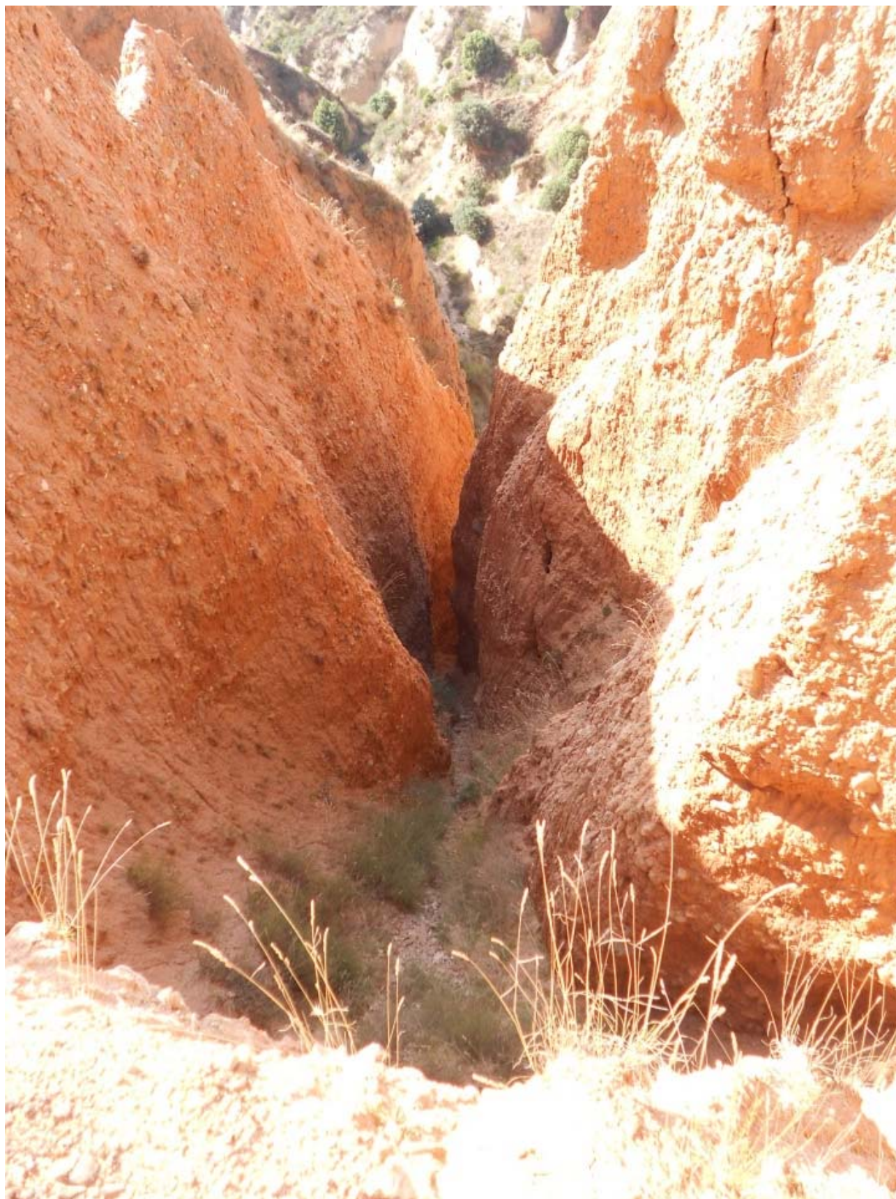
Figura o Foto 18: Cárcava del Cerro Negro. Callejón.
