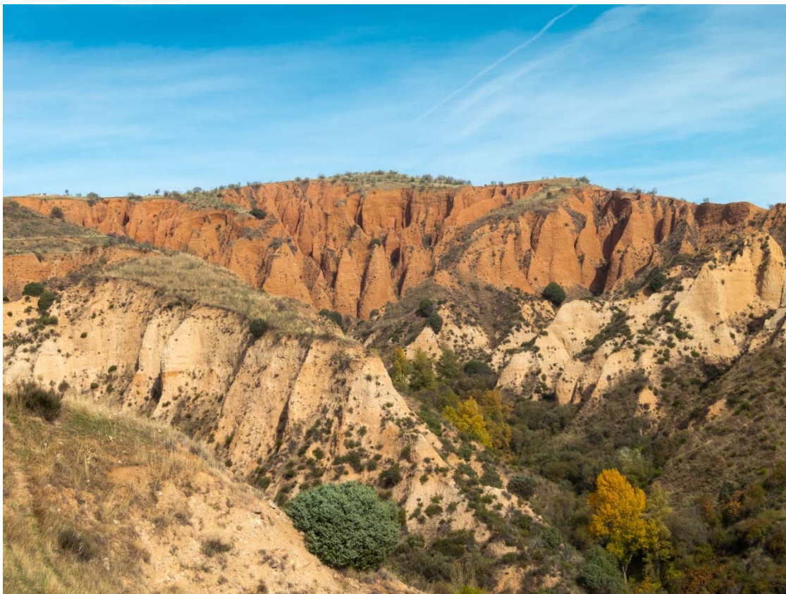
Figura o Foto 27: Cárcava del Cerro Negro vista desde el Sector Occidental.
