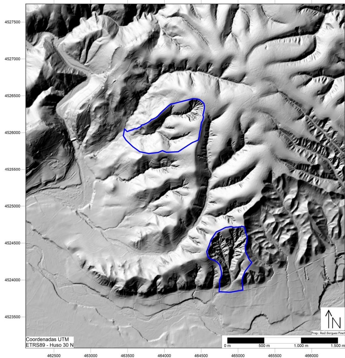
Figura o Foto 2: Ubicación de los Sectores sobre Mapa de Relieves Sombreados.
