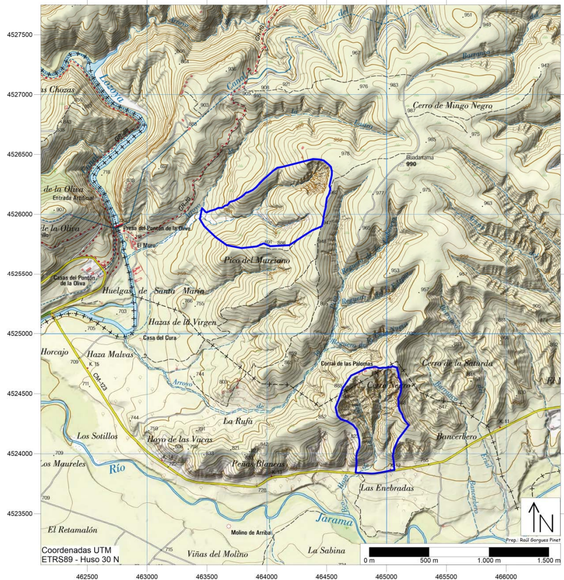
Figura o Foto 1: Ubicación de los Sectores en el Mapa topográfico.
