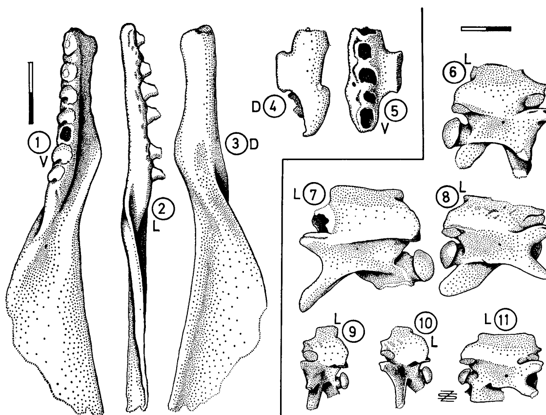
Fig. 11.—Serpentes indet. 1-3, left pterygoid (MNCN, no Alg I-59); 4, 5, posterior fragment of right maxilla (MNCN, no Alg I-60); 6, cloacal vertebra (MNCN, no Alg I-61); 7, mid-caudal vertebra (MNCN, no Alg I-62); 8, posterior caudal vertebra (MNCN, no Alg I-63); 9, cloacal vertebra (MNCN, no Alg I-64); 10, anterior caudal vertebra (MNCN, no Alg I-65); 11, posterior caudal vertebra (MNCN, no Alg I-66). D - dorsal, L - lateral, V - ventral views. Scale equals 2 mm.
