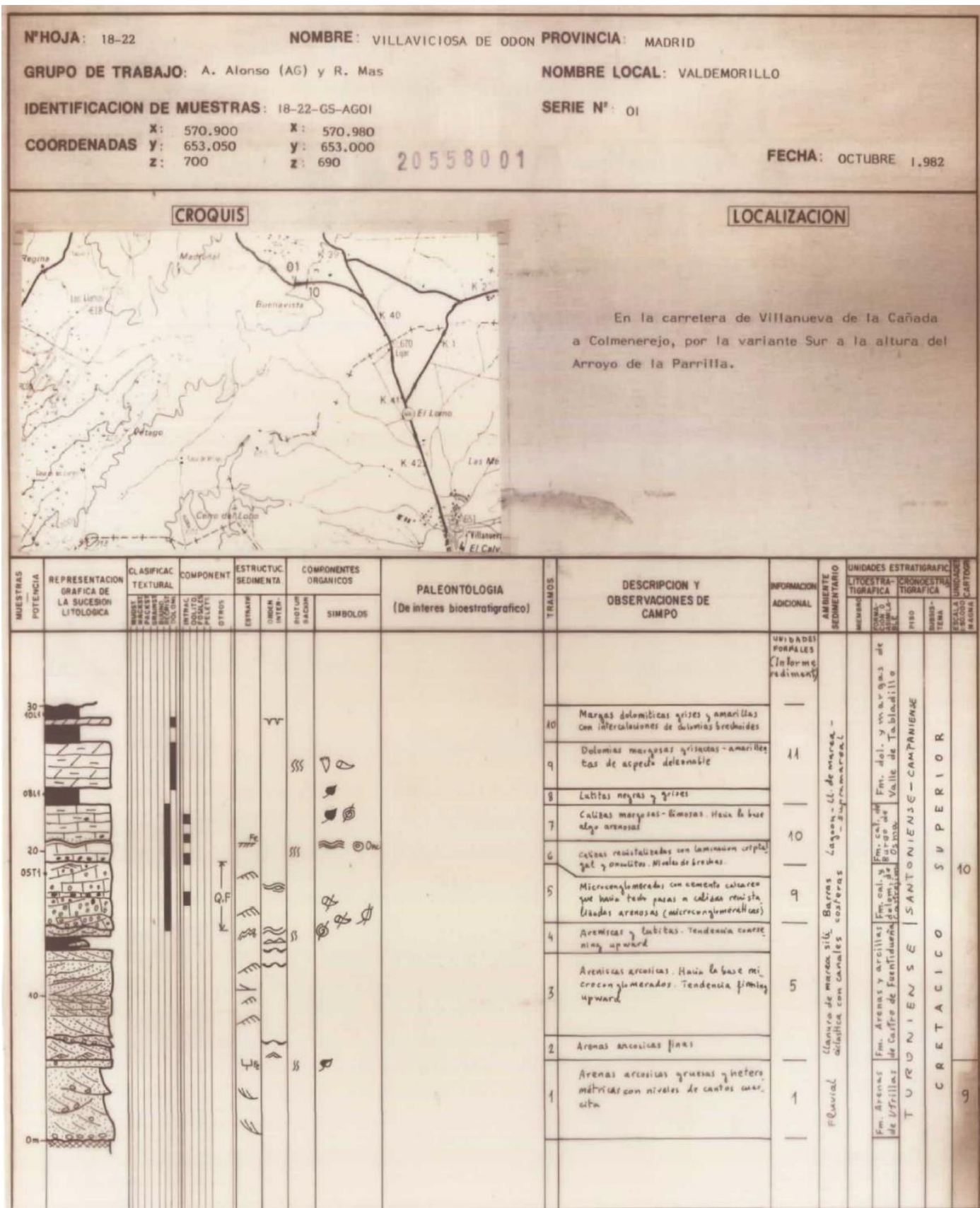
C-TM012-01. Columna estratigráfica del Cretácico de Valdemorillo incluida en el Informe Sedimentológico (Alonso y Mas 1982) de la Documentación Complementaria de la hoja MAGNA 558 (Majadahonda) (Portero et al. 1990). El Miembro Valdemorillo está formado por los tramos 1, 2, 3 y 4 (Unidades Formales del Informe nºs 1 y 5)
