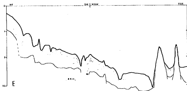
Fig. 4. Perfil sísmico Air-gun (0,7 litros) realizado oblicuamente al talud catalán, para luego atravesar normalmente la depresión de Valencia. En la primera parte aparecen los cañones submarinos que entallan el margen continental, sin alcanzar al substrato del Mioceno; en la depresión de Valencia y junto al valle central, se elevan dos pitones volcánicos que atraviesan y alteran la disposición del relleno sedimentario. M = Messiniense.
