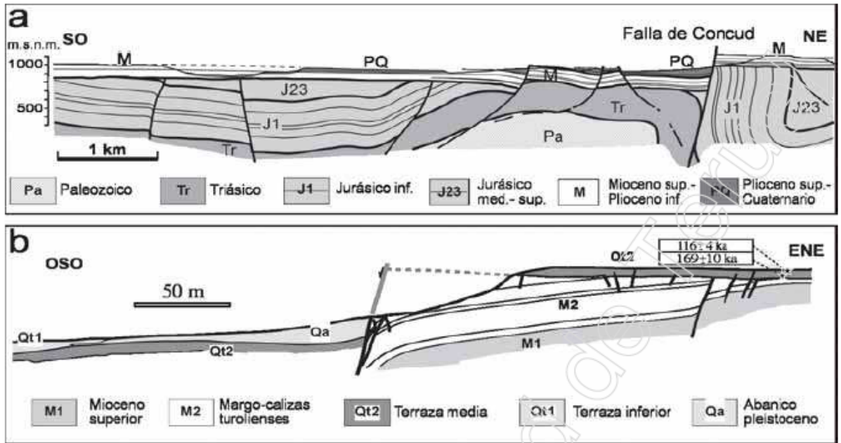
Fig. 1 Cortes geológicos de la falla de Conchud
