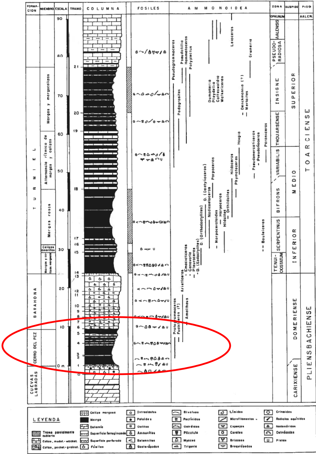
FIG.- 6. COLUMNA ESTRATIGRAFICA DEL GRUPO ABLANQUEJO EN TURMIEL
