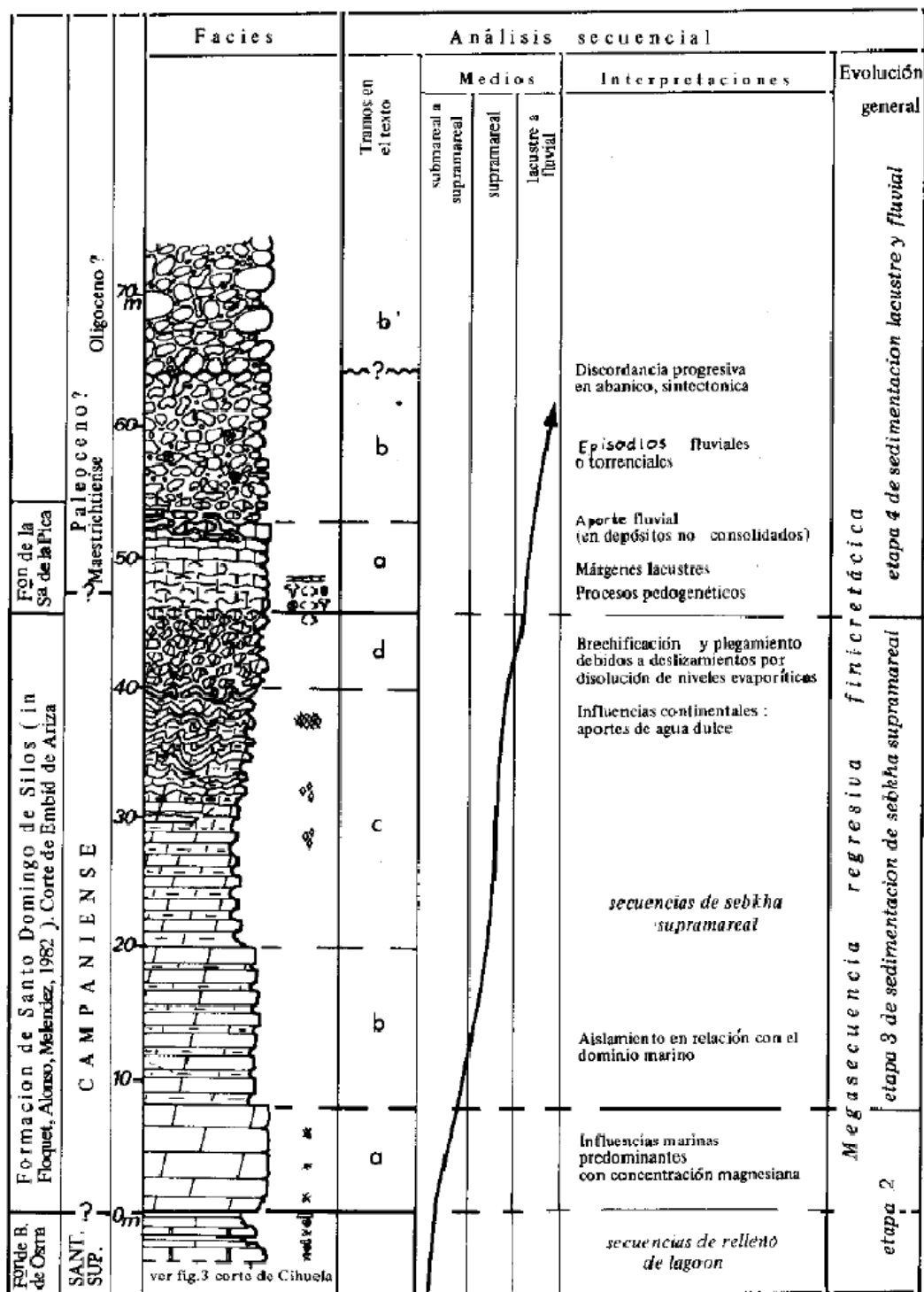
FIG. 4.—Corte de Embid de Ariza (Lat.: 41° 23' - Long.: 1° 43'). Etapa 3 de sedimentación de sebkha supramareal (Campaniense), y etapa 4 de sedimentación lacustre y fluvial (Campaniense superior?, Maestrichtiense a Paleoceno?) en la megasecuencia regresiva finicretácica; según Floquet, Meléndez, Pedayúé (1981).
