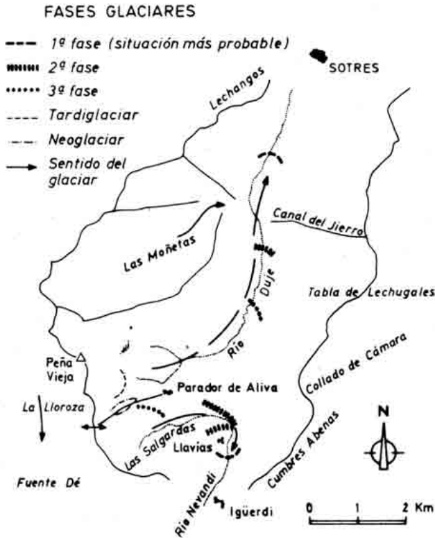
Fig. 4. Esquema de evolución de los diferentes momentos glaciares. Se distingue la glaciación principal con sus tres fases (1ª: expansiva, 2ª: estabilización y 3ª: retroceso) y, muy probablemente, las más recientes (Tardi y Neoglaciario). Asimismo, se consignan los flujos de los valles principales.
