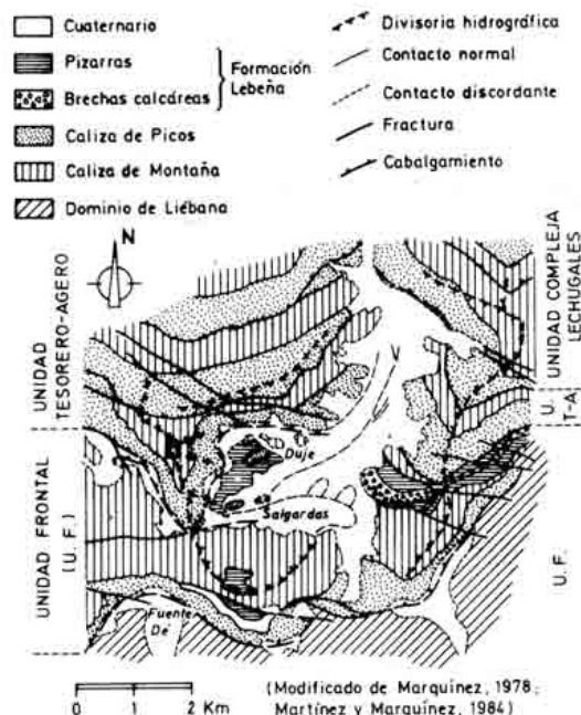
Fig. 2. Esquema Geológico.
