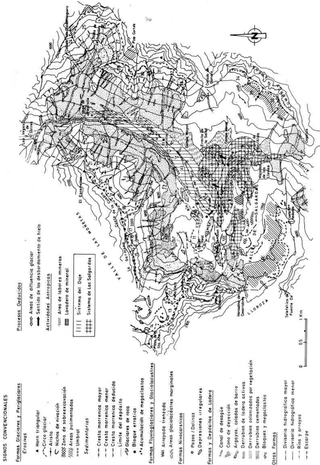
Fig. 3. Mapa morfológico de los puertos de Aliva. Fig. 3. Morphologic map of the Aliva.
