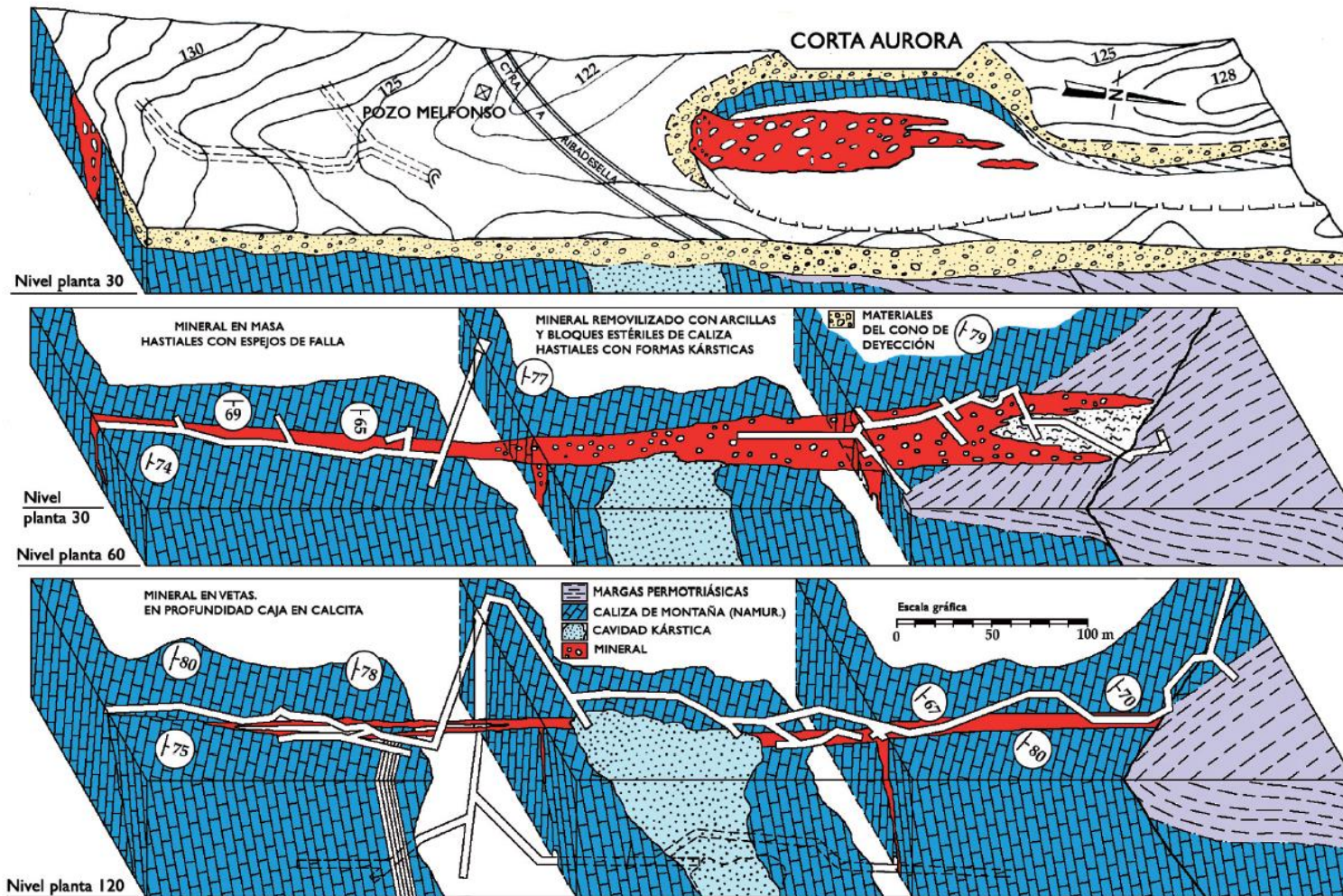
Bloques diagrama del filón-capa Aurora y sus explotaciones (corta Aurora-Pozo Melfonso). Datos de Tejerina & Zorrilla (1980).
