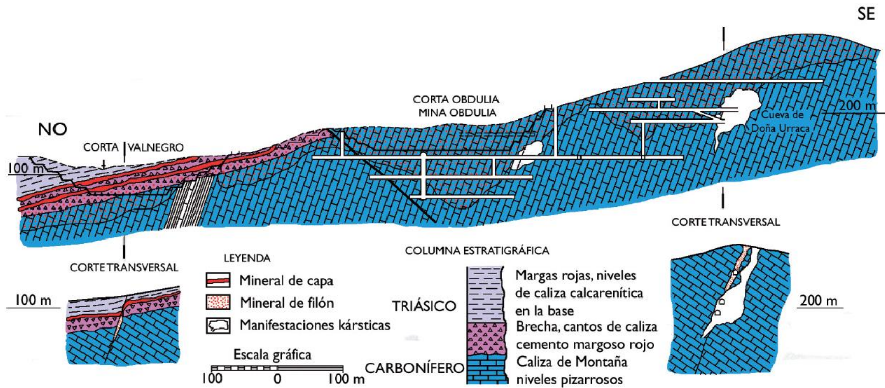
Sección longitudinal (y transversal) de la mineralización del filón Obdulia (mina Obdulia-Corta Valnegro). Datos de Tejerina & Zorrilla (1980).
