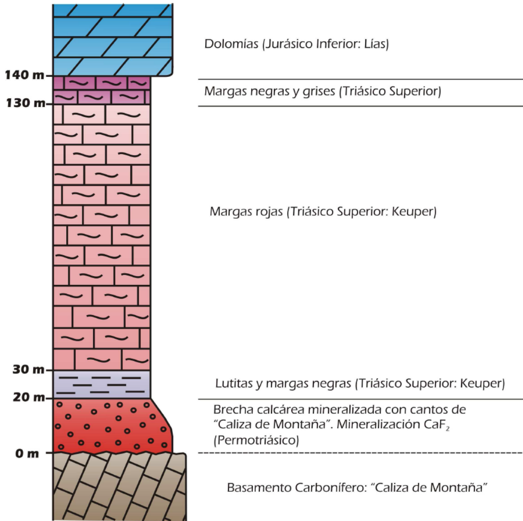
Columna estratigráfica genérica en la mina Emilio (según Sánchez, 2009)
