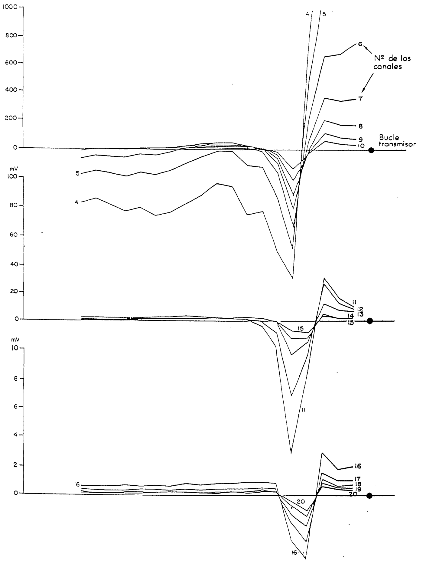
Fig. 8 - Ejemplo de anomalía originada por un conductor
