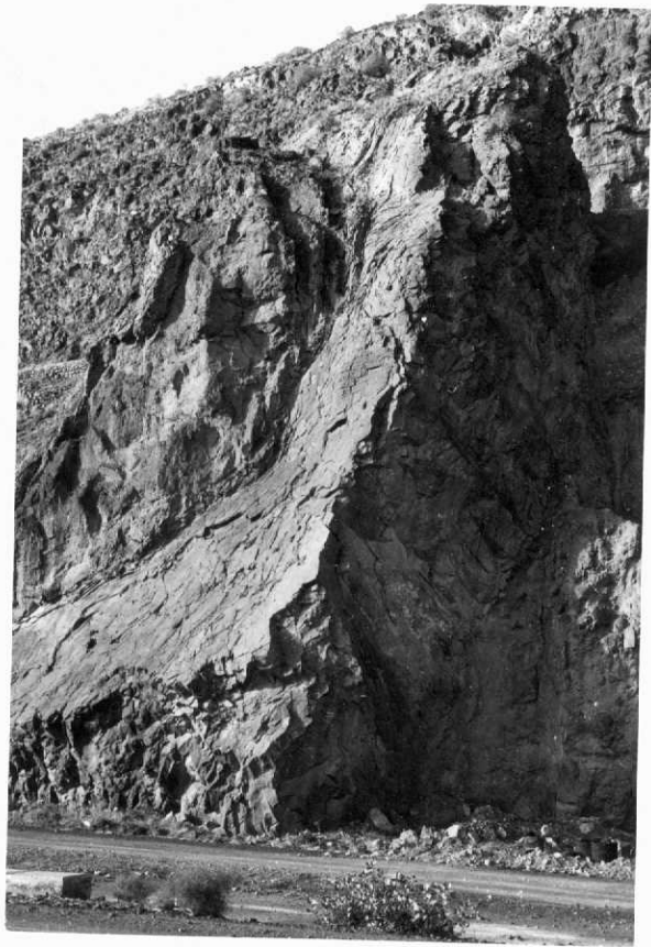
39-39-AD-CG-1938.- Potente dique basáltico atravesado piroclastos de la Serie I.
