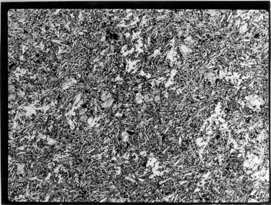
39-39-AD-VA-1336.- LN x 5. Fotomicrografía de basalto micropor o f ídico. Microcristales de augita en matriz de microlitos pla g - gioclásicos con cierta orientación fluidal.
