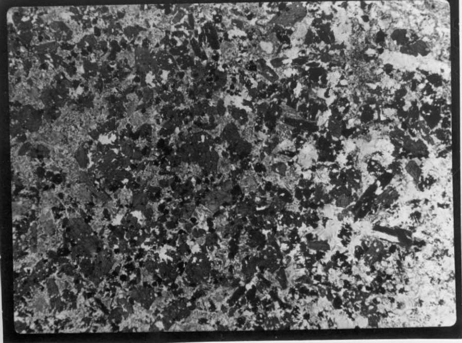
39-39-AD-VA-1382.- LN x 5. Fotomicrografía de enclave máfico en pitón fonolítico. Textura gabroidea. Cristales de anfíbol, augita egirínica, plagioclasa y carbonatos secundarios.
