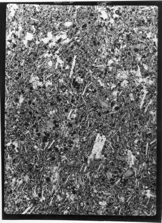
39-38-AD-VA-16.- LN x 9 Basalto augítico plagioclásico. Detalle de la textura. Se aprecian fenocristales de plagioclasa y augita. Matriz con pequeños olivinos iddingsitizados. Fotomicrografía.
