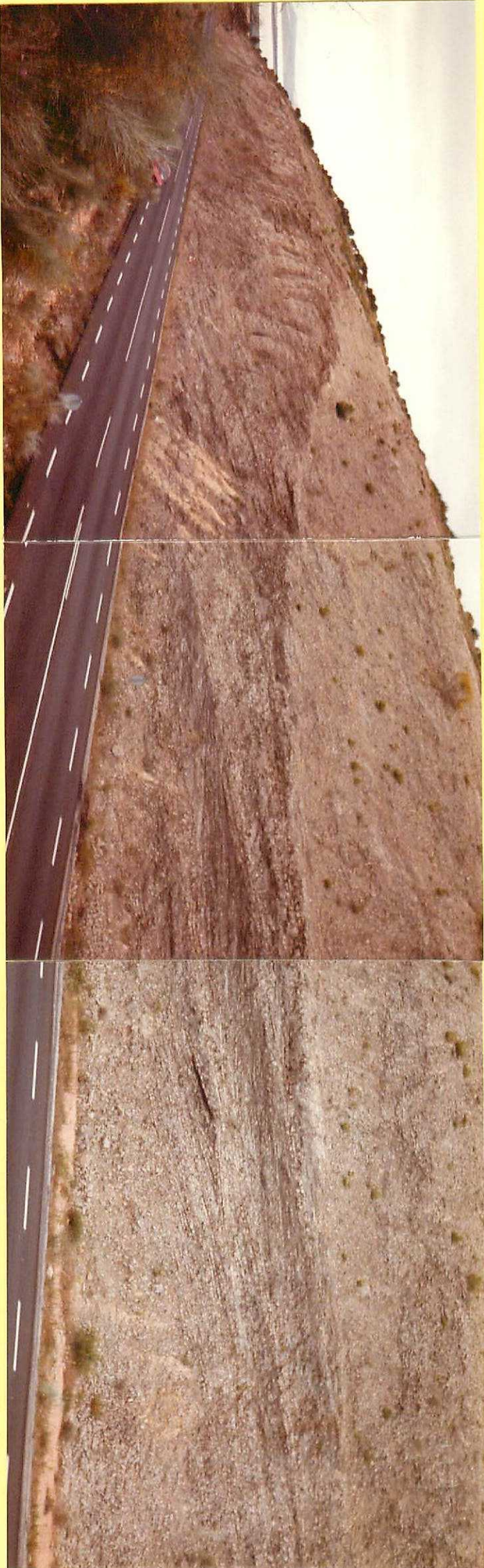
Fot. 3.- Cra. de Bornos a Aras de la Frontera. Biocalcarenita miocena. Hoja de Montellano. Afloramiento próximo a la columna 20. Unidad cartográfica 24. Los cosets de estratificación cruzada se superponen sin intercalaciones pelíticas.
