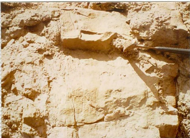
16-41-IB-AS-9508.- Detalle del mismo banco turbidítico con laminación cruzada en la parte superior -- (intervalo C) y paralela (b)).
