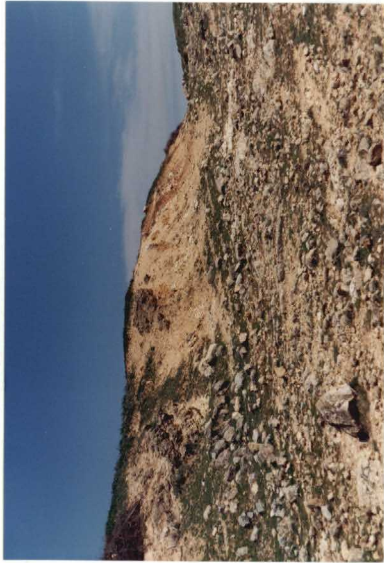
FOTO 22-27-AD-AG-9314 F.- Depósitos mixtos en las facies del Cretácico superior (Campaniense) en las proximidades de Carrascosa de Haro.
