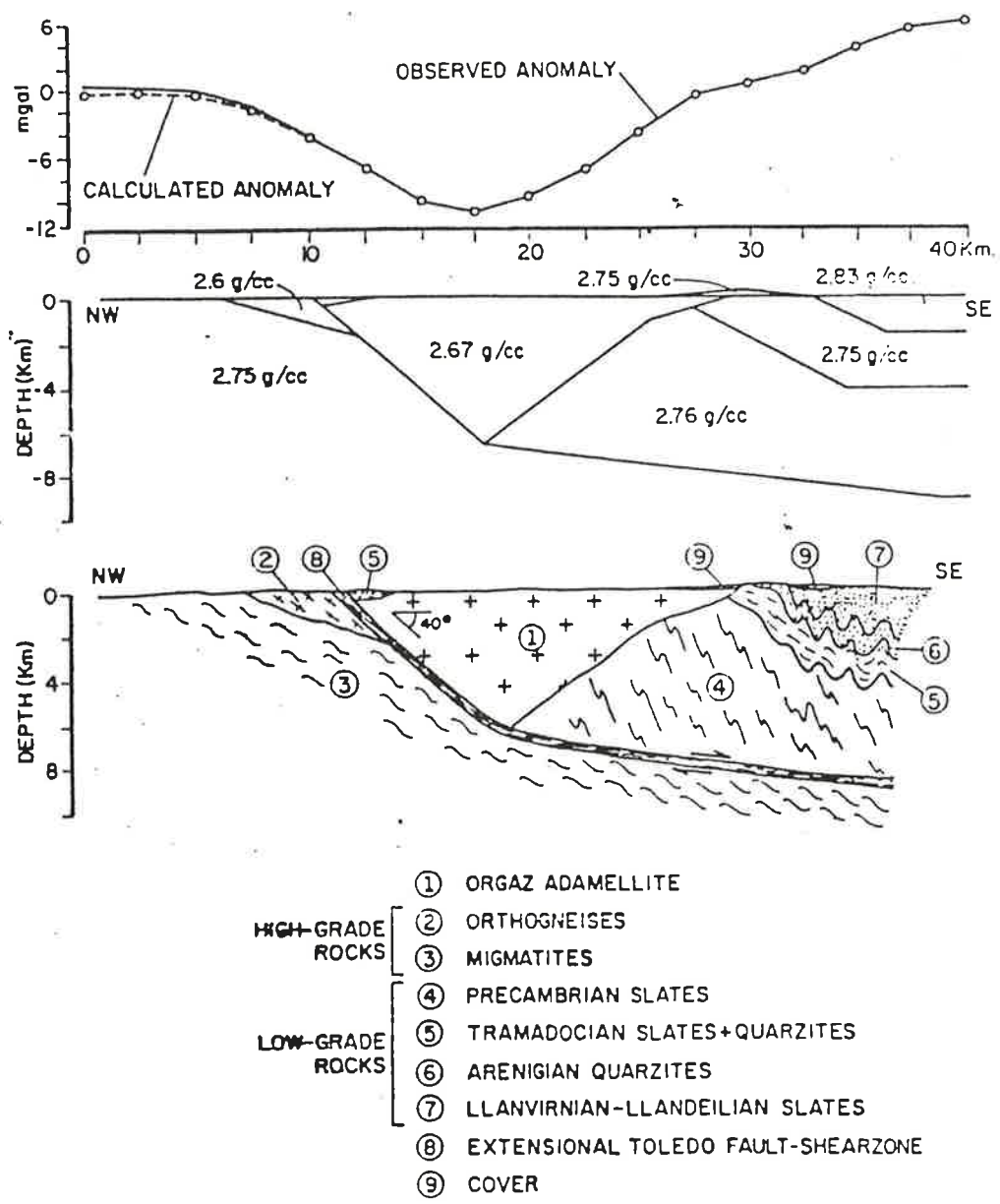
FIGURA 1.- Corte geológico interpretativo del Granito de Orgaz (parte oriental de la alineación Plutónica Mora-Gálvez) a partir de datos gravimétricos (según CASQUET et al., 1988; basado en SANTA TERESA et al., 1983).
