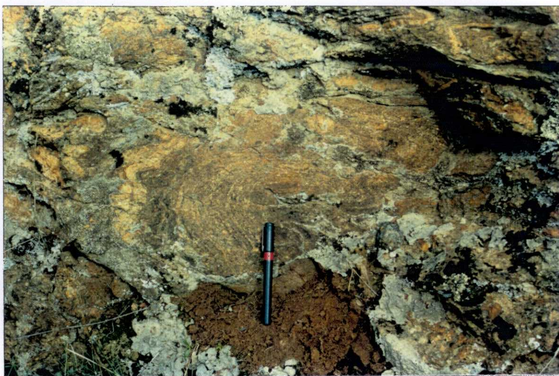
MP- 9415.- Metasedimentos con la foliación principal ( S_2 ) plegada por pliegues de D_3 . Al SO. de Pepino.
