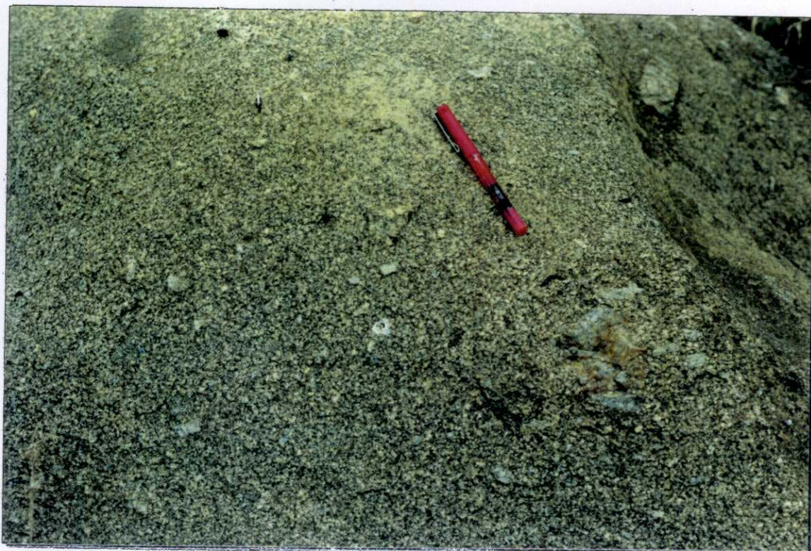
MP- 9413.- Agregado globular de cuarzo en granitoide anterior (7). Al S. de Cervera de los Montes.
