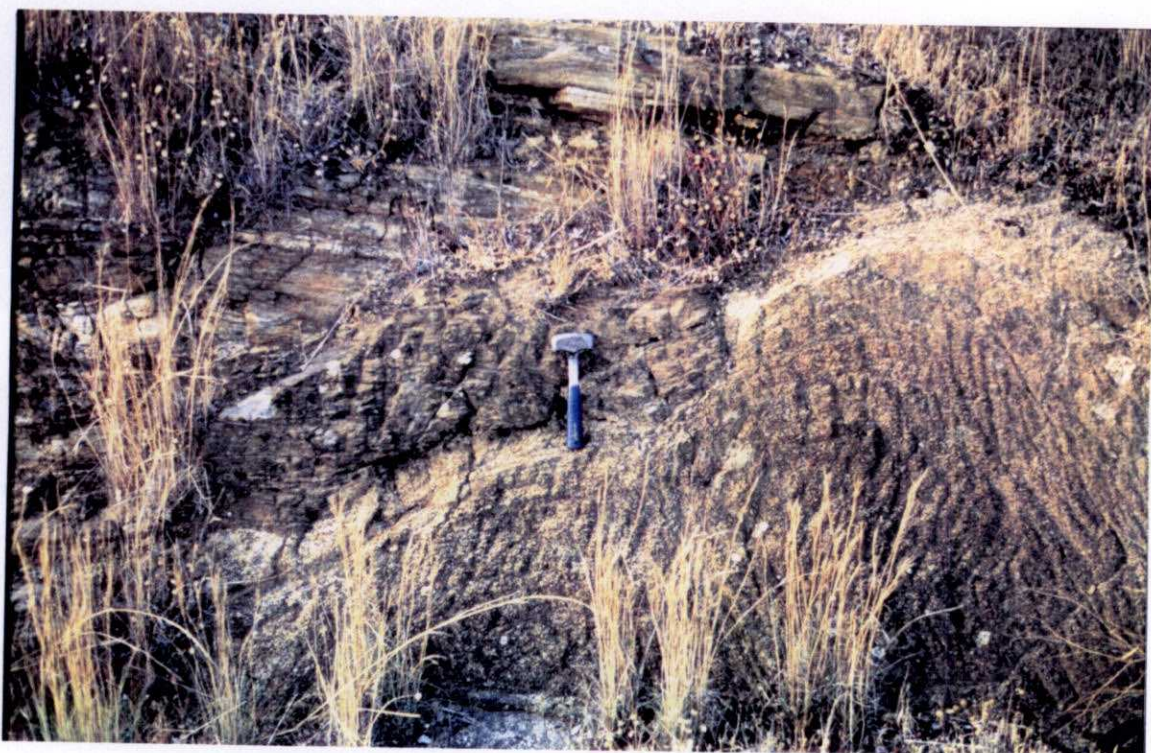
MP- 9403.- Contacto intrusivo entre adamellita biotítica ± moscovita de grano medio-grueso con megacristales (11) y metasedimentos (15). Al N. de Hinojosa de San Vicente.
