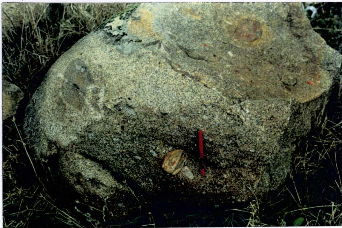
MP- 9412.- Enclaves metasedimentarios en adamellititas biotíticas \pm moscovita \pm cordierita de grano fino-medio con megacristales (7). Al S. de Cervera de los Montes.
