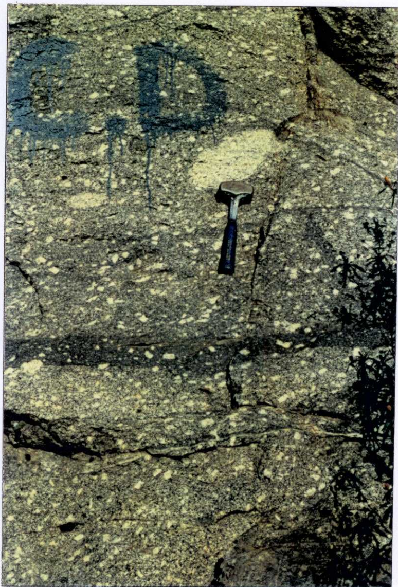
MP- 9410.- Adamellita biotítica \pm moscovita de grano medio-grueso porfídica (11), con enclaves de leucogranitos foliados, afectada por una banda de ultramilonitas frágil-dúctiles. Zona de Cizalla de San Vicente. Carretera de El Real de San Vicente a Navamorcuende.
