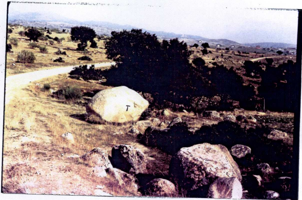
MS- 9235.- Gran bloque leucogranítico en el Cerro Pendón. Unidad con grandes bloques (20).
