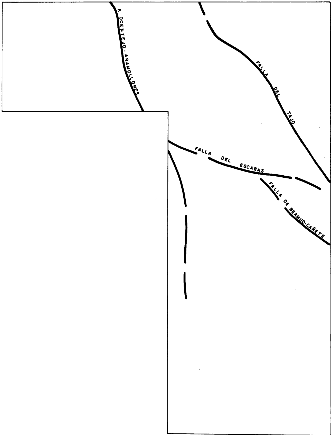
FIGURA 2.- FALLAS y LINEAMIENTOS DE ZOCALO
