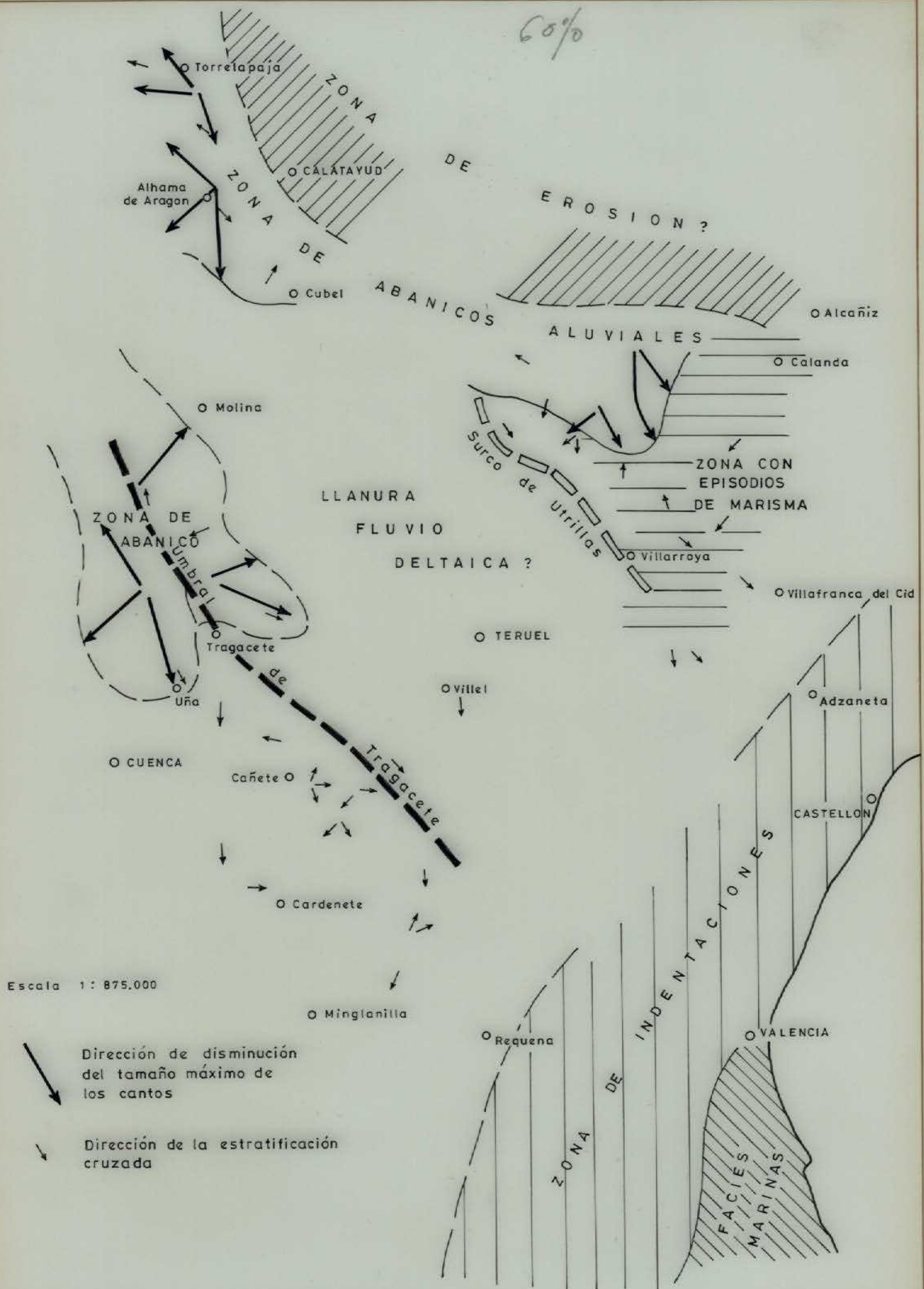
Fig MAPA PALEOGEOGRAFICO DURANTE EL ALBENSE Basado en datos de SAEFTEL ( 1.961 )
