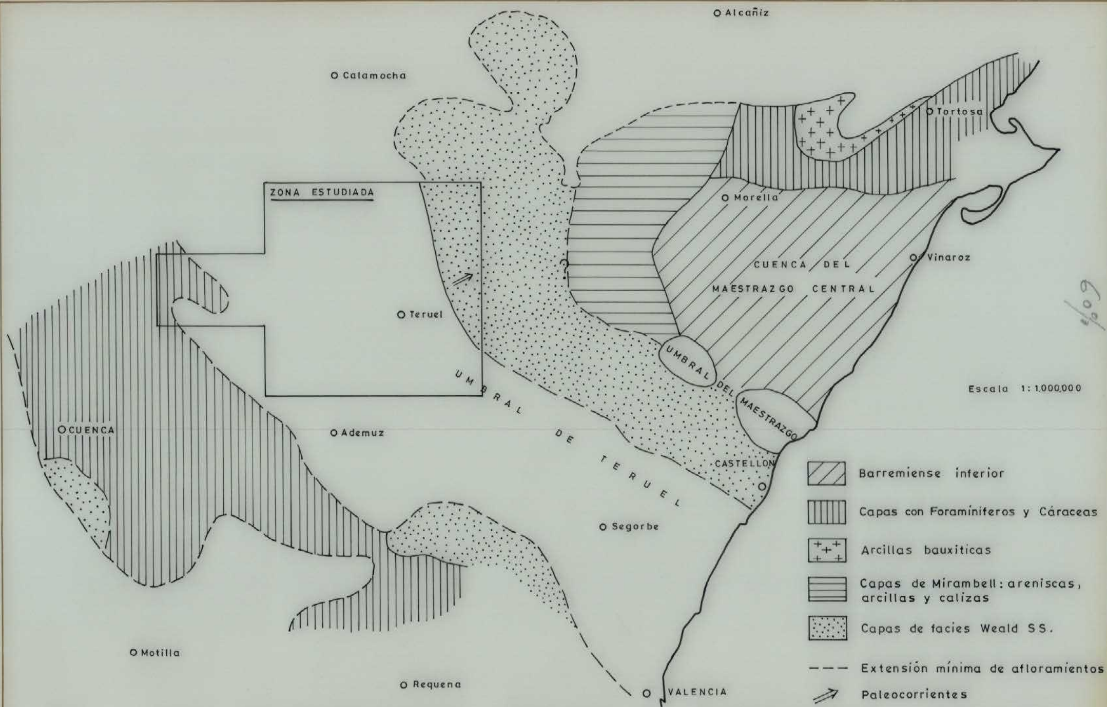
Fig. MAPA PALEOGEOGRAFICO DURANTE EL BARREMIENSE INFERIOR Según Canerot (1975) Viallard (1972), modificado
