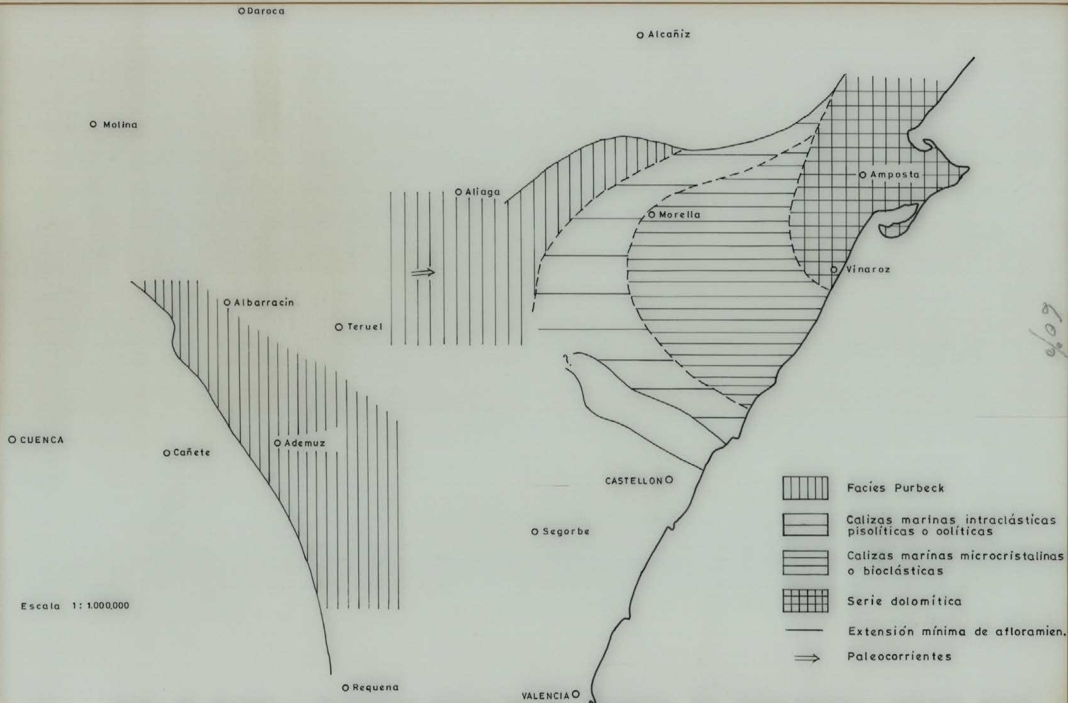
Fig. MAPA DE FACIES Y EXTENSION MINIMA DE LOS TERRENOS DEL PORTLANDIEN. - CRETAC. BASAL Datos de Viallard, Canerot y propios
