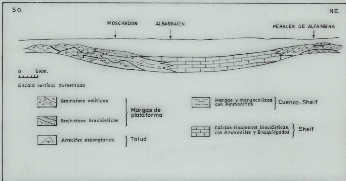
Esquema deposicional en el Bajociense superior - Bathoniense
