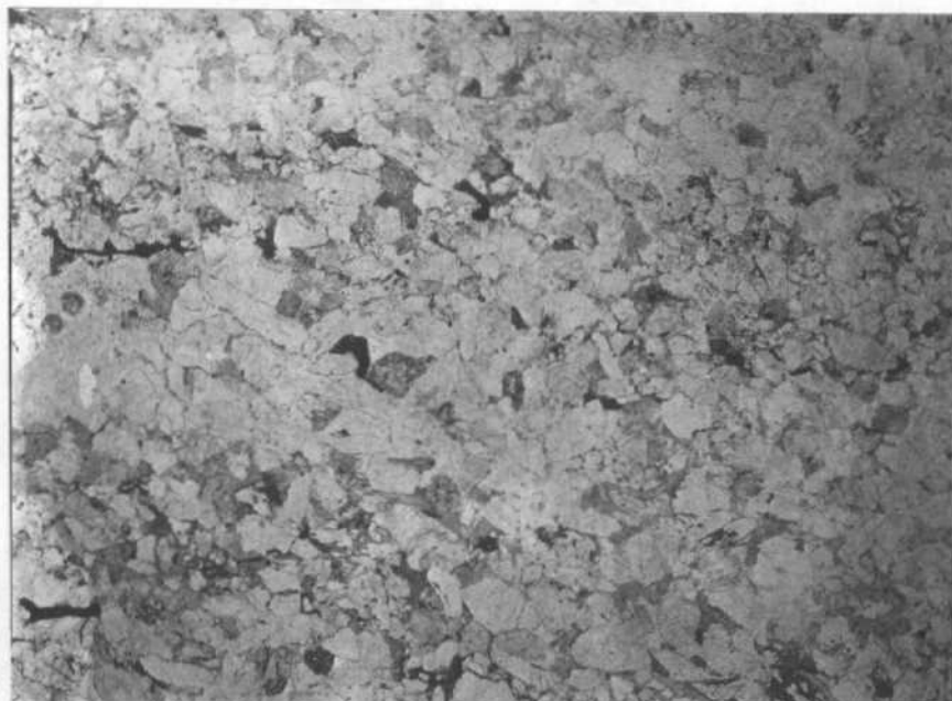
FOTO 3 (23-19-FM-4006) x 12 Arenisca (subarcosa) con cemento ferruginoso y matriz sericitica. Depósito terrígeno. BUNTSANDSTEIN
