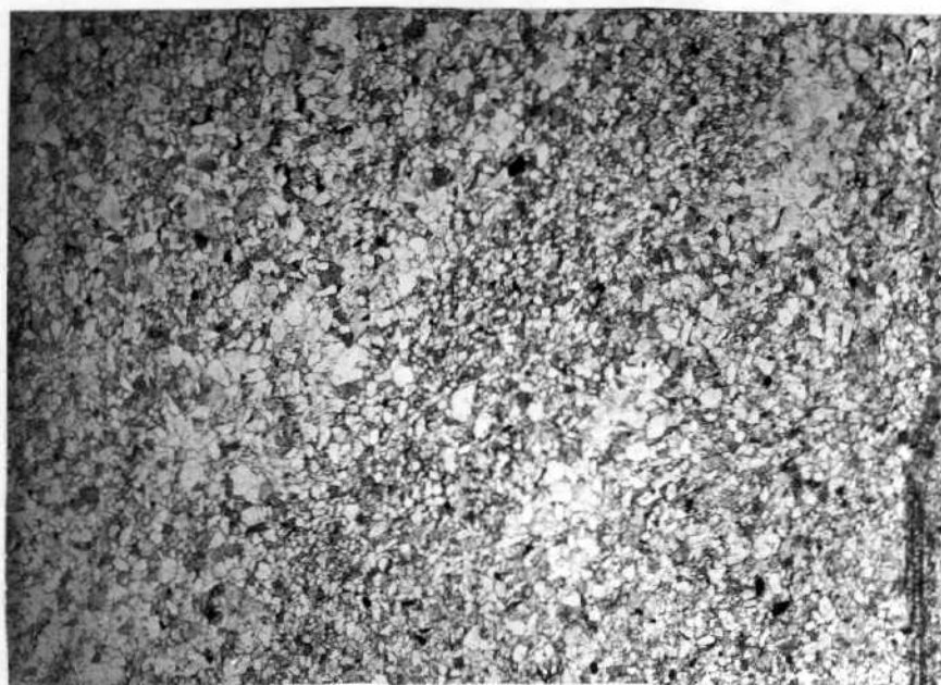
FOTO 4 (25-21-MT-5174) Arenisca arcillosa (subarcosa) con matriz sericitica. Depósito terrígeno. BUNTSANDSTEIN
