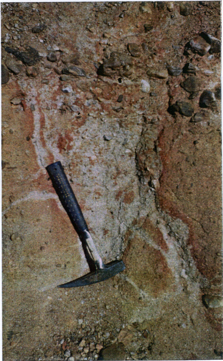
Foto 17. Afloramiento arcósico en el Apeadero de Villares de Yeltes con fuertes rasgos de hidromorfía
