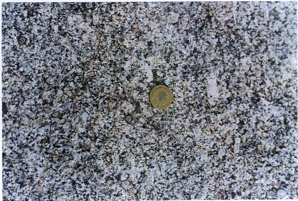
Foto 8. Granodiorita de Bañobárez. Facies con grano grueso y cristales porfídicos de feldespato de distribución esporádica
