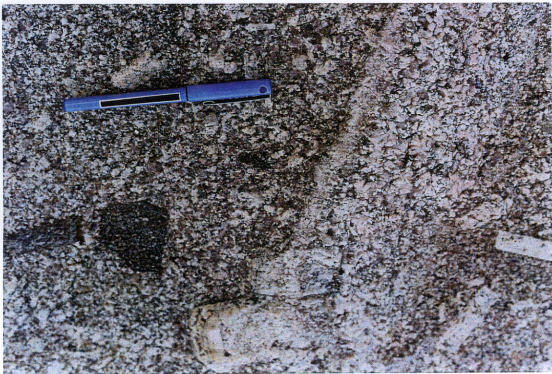
Foto 6. Granodiorita de Bañobárez con megacristales de feldespato tabulares, un diquecillo pegmoaplítico y enclaves microgranudos (facies tonalíticas)
