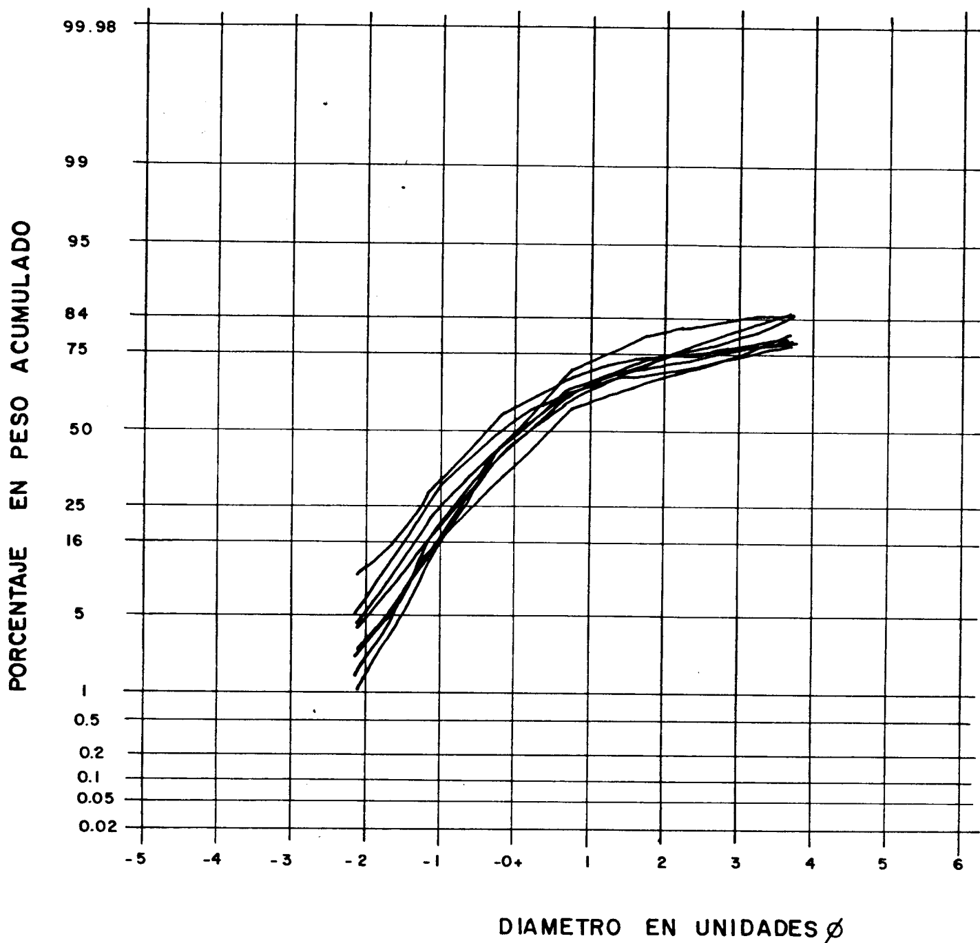
Curvas granulométricas. Facies deGarciahernandez.
