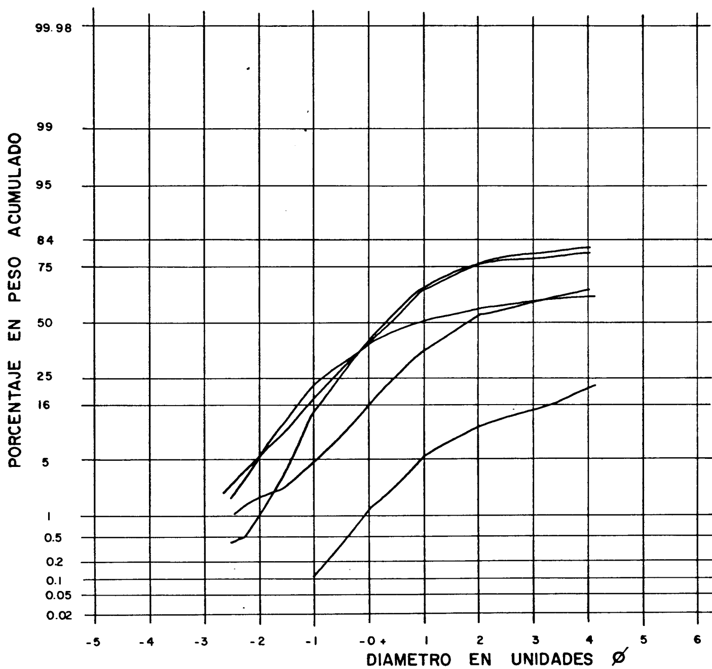
Curvas granulométricas. Facies de Cilloruelo.
