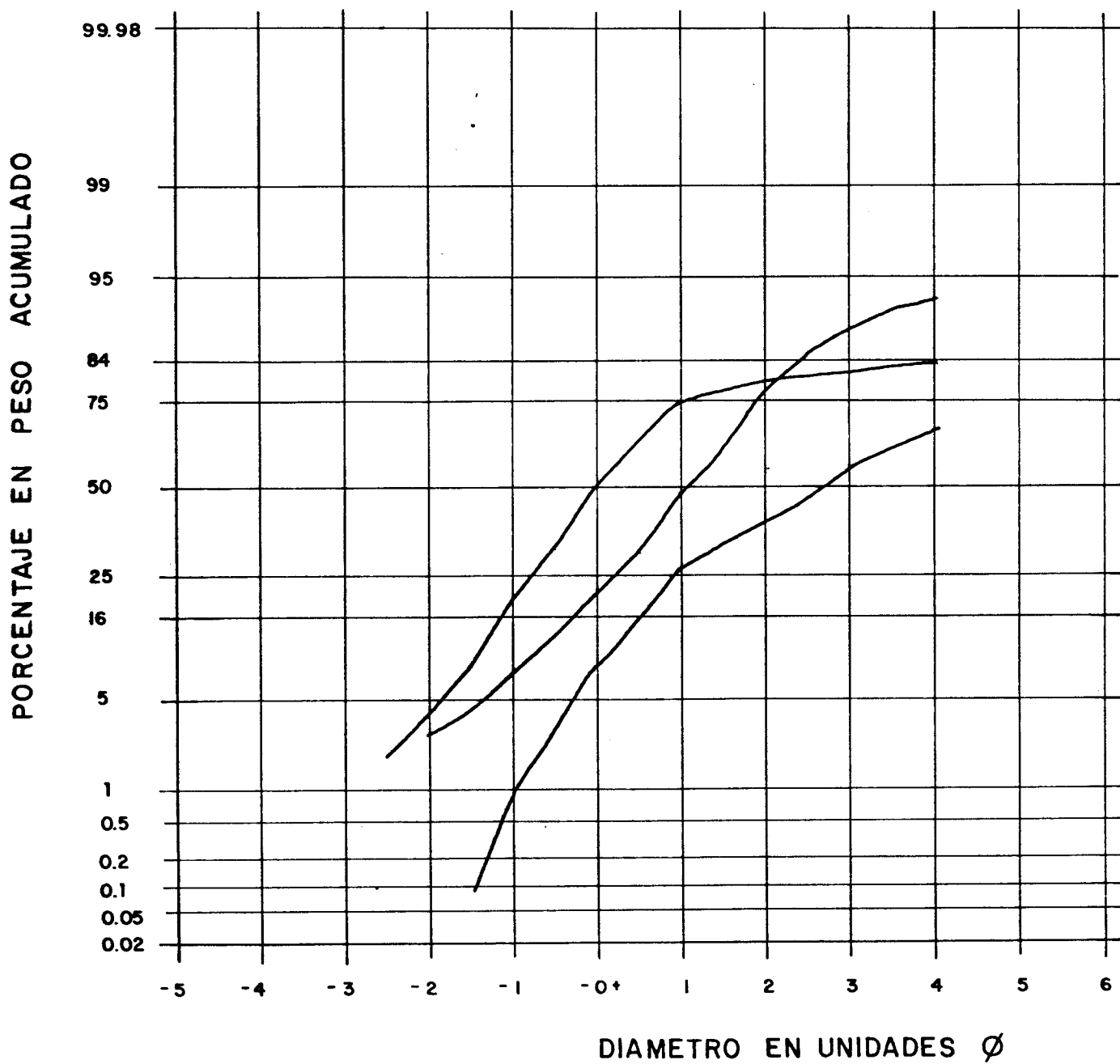
Curvas granulométricas. Formación Areniscas de Salamanca.
