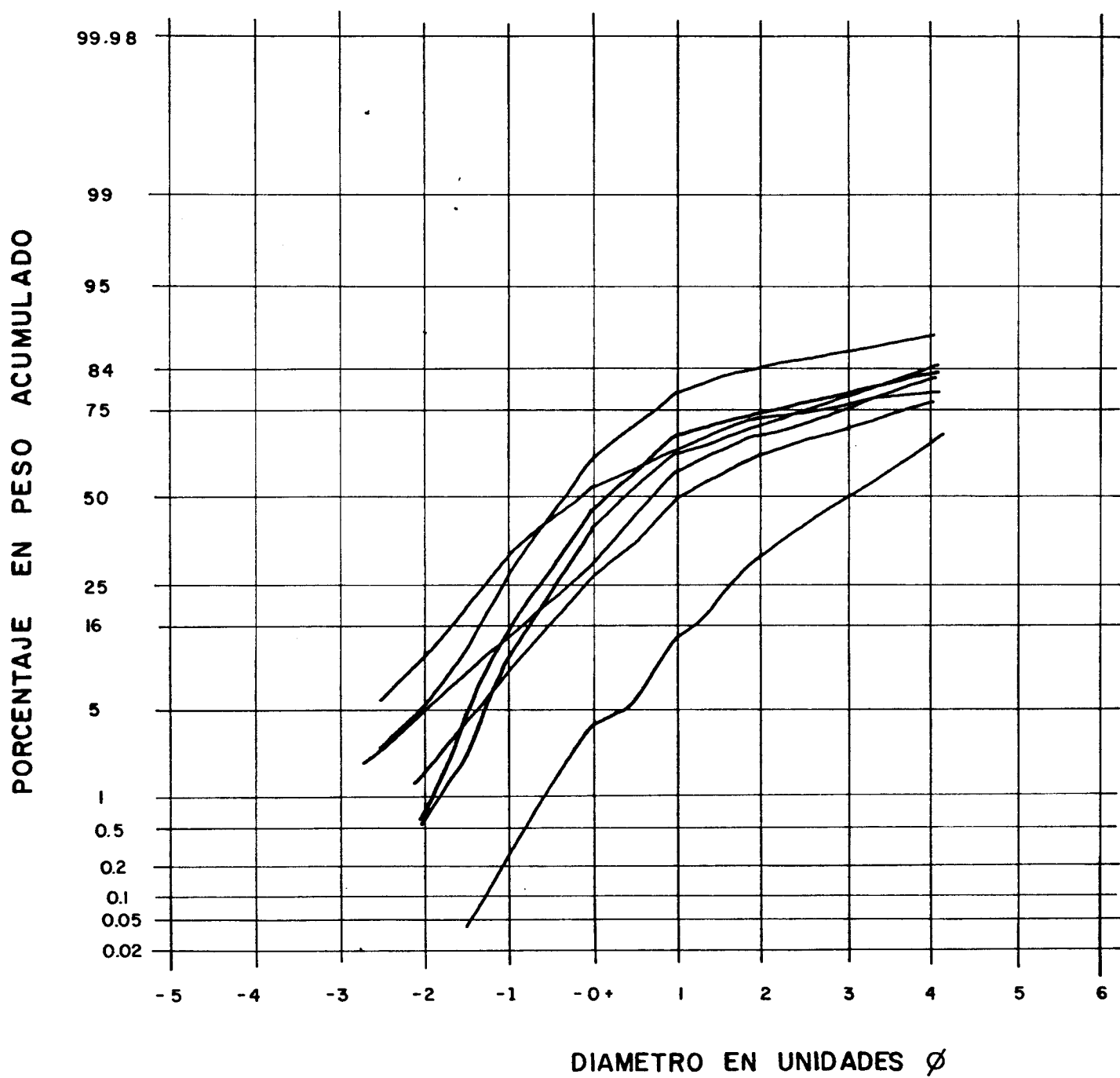
Curvas granulométricas. Facies de Amatos.
