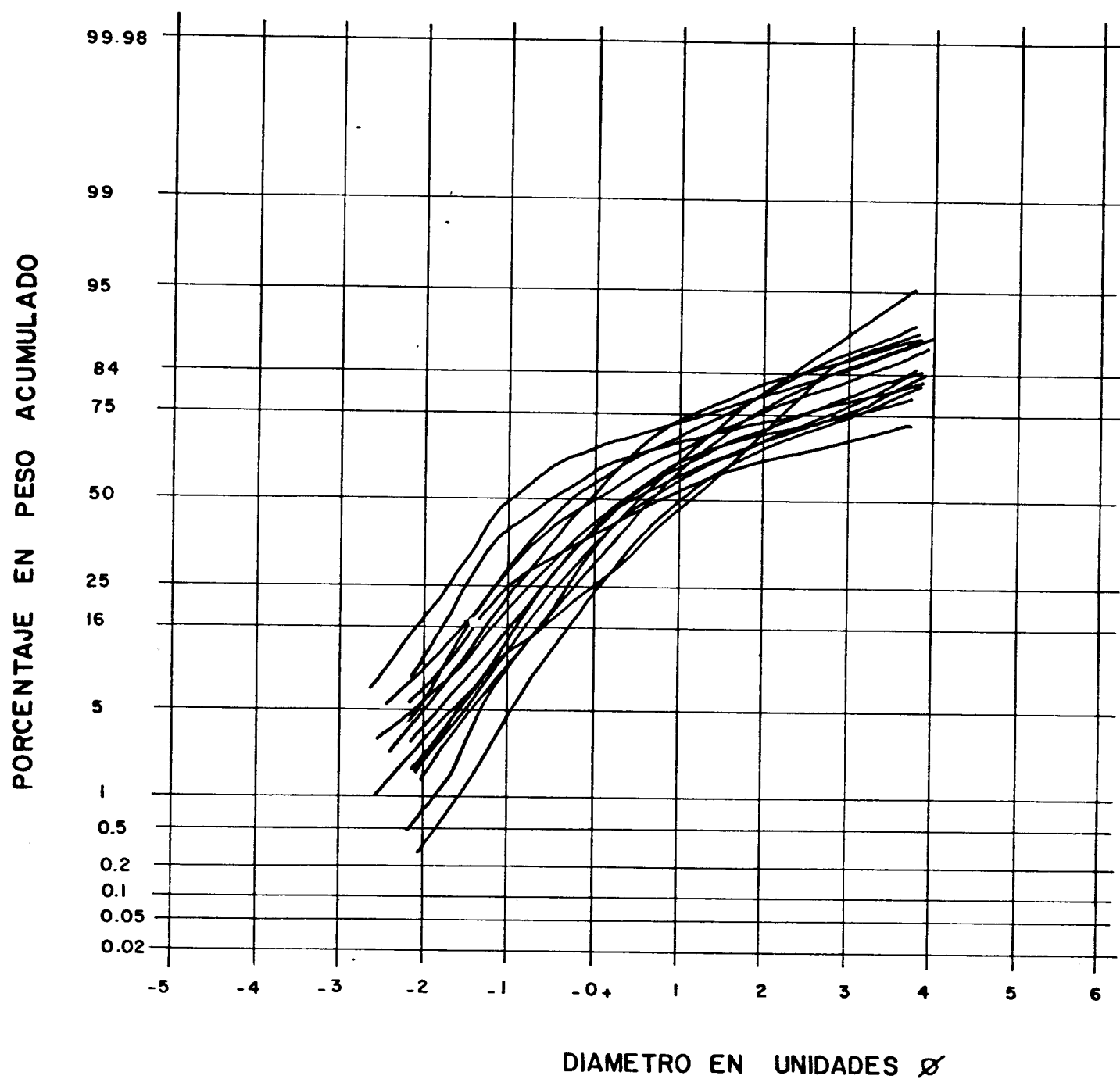
Curvas granulométricas. Facies de Garcíhernandez.
