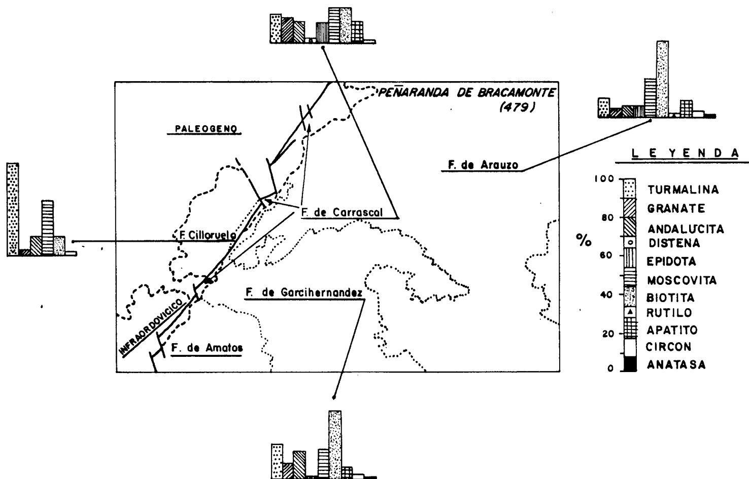
MINERALES PESADOS DE LAS FACIES MIOCENAS
