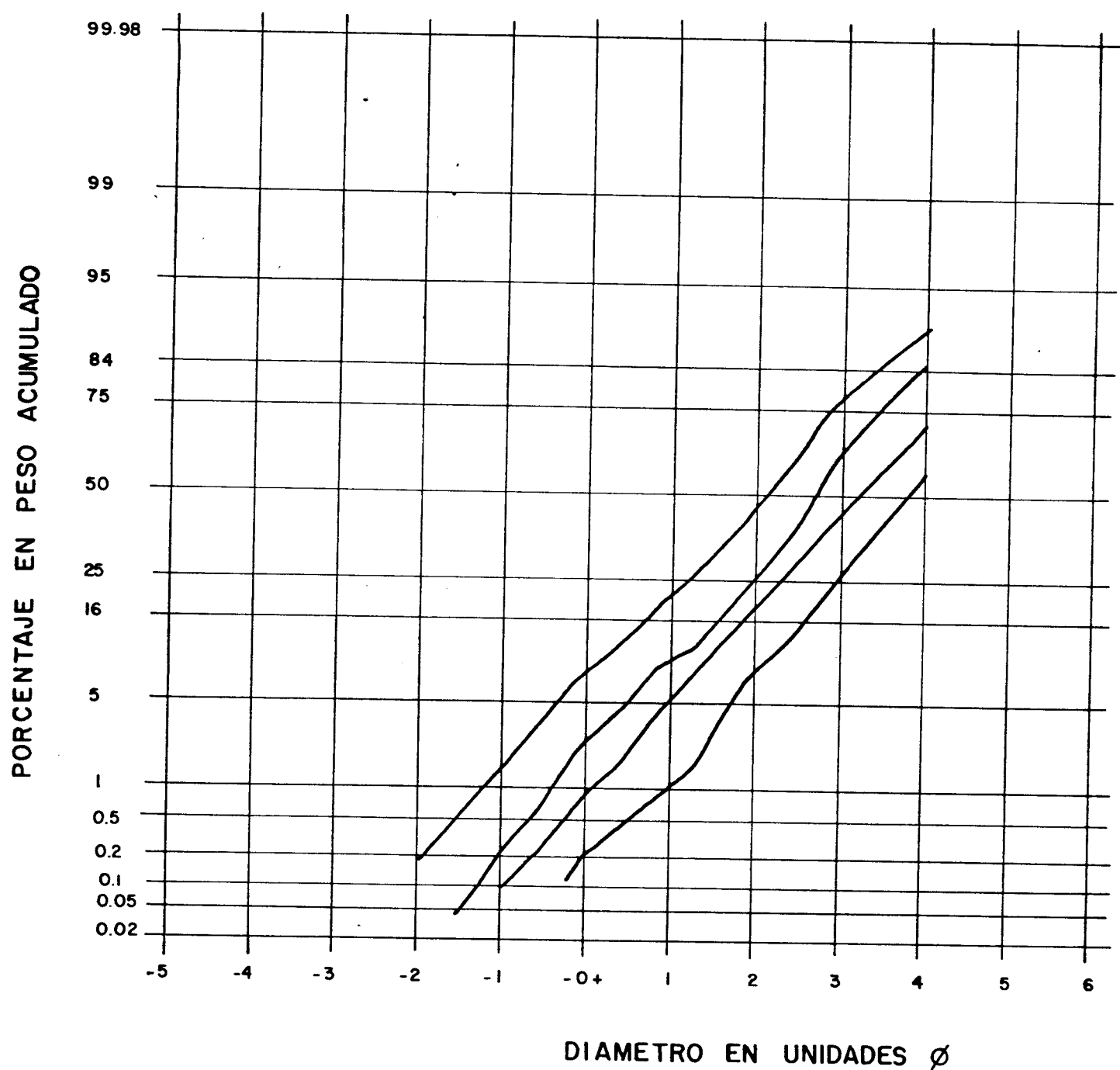
Curvas granulométricas. Facies de Carrascal.
