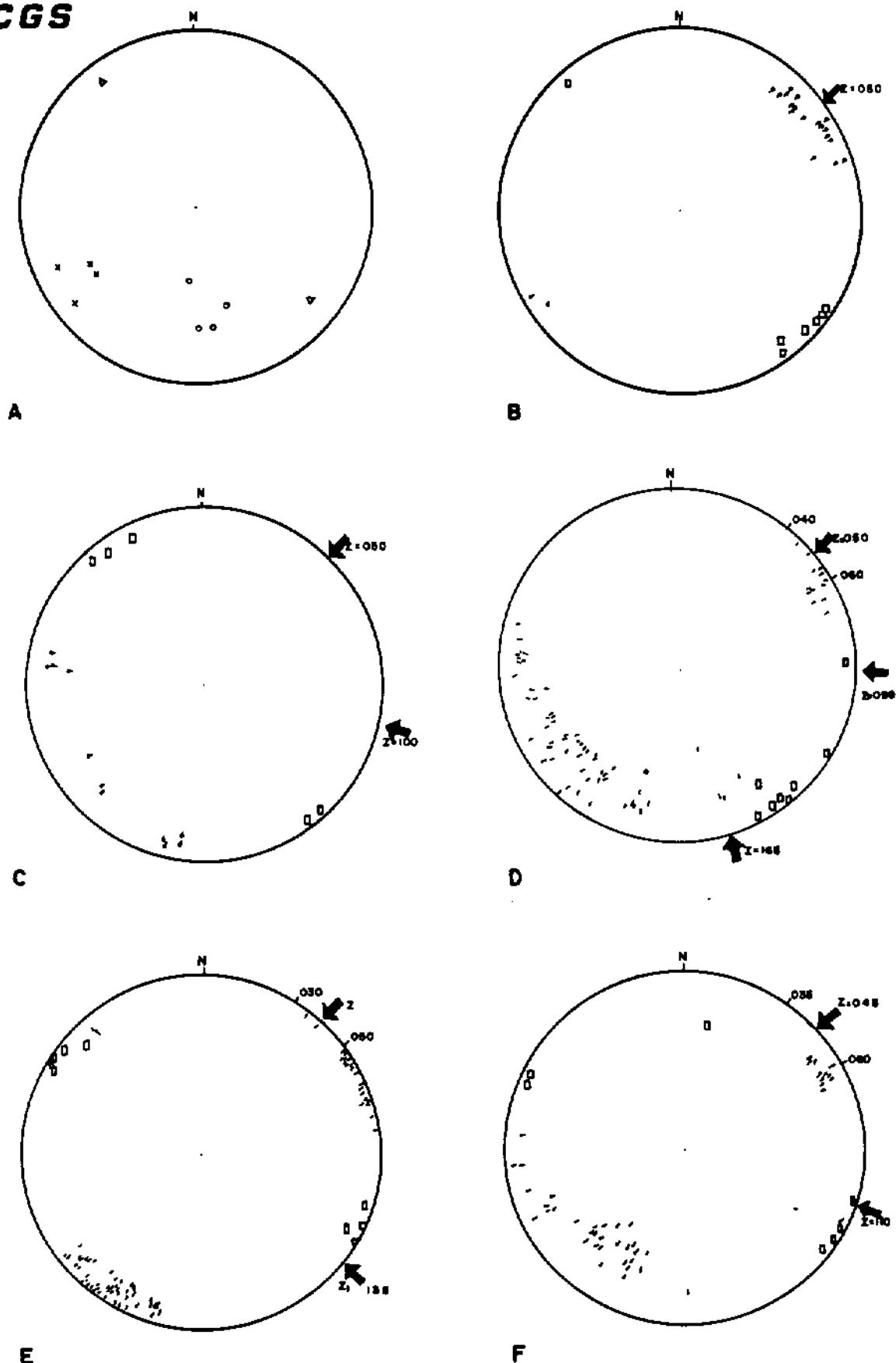
FIGURA 4.- ANALISIS MICROTTECTONICO. Orientación de los elementos microestructurales del Paleozoico de Cueva del Hierro (A). (Círculos, ejes de pliegues; cruces, polos de la esquistosidad; trinagulos: lineación de intersección So-S1). Estilonolitos (puntos) y grietas de tracción (cuadrados) en los materiales jurásicos y cretácicos de las hojas de Peralejos (B), Valdeolivas (C), Fuertescusa (D), Las Majadas (E) y Cuenca (C).
