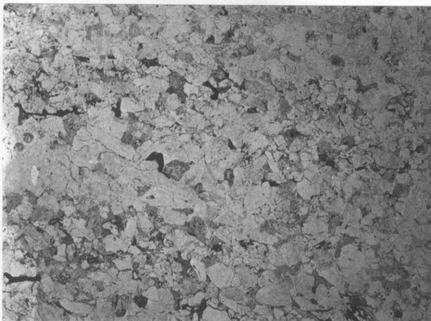
FOTO 3 (23-19-FM-4006) x 12 Arenisca (subarcosa) con cemento ferruginoso y ma- triz serícitica. Depósito terrígeno. BUNTSANDSTEIN
