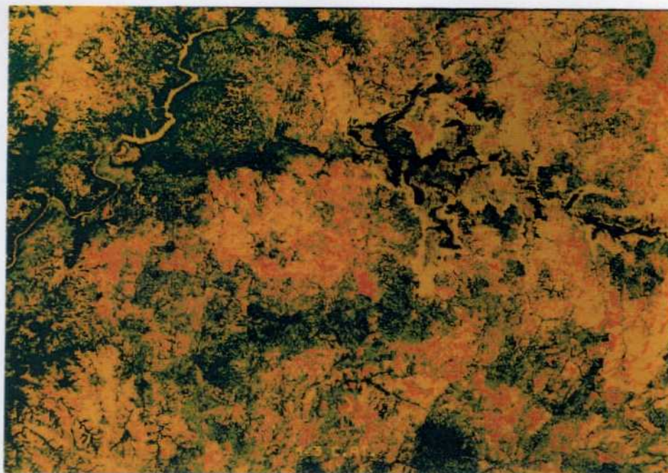
fig.1. Segmentación de números digitales en el cociente entre las bandas thematic mapper 4 y 3. Colores asignados a valores de bajos a altos, que corresponden a zonas con densidad de recubrimiento vegetal proporcional: amarillo, naranja, verde claro, verde oscuro. Hoja de Fermoselle.
