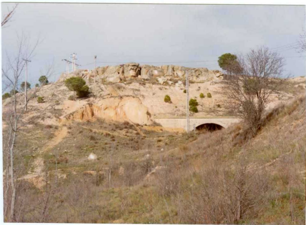
13-15 -GM-AC -505 .- Arenisca con niveles de grava ( T_{C.1-2}^{A-Aa} ) sobre las que yacen las areniscas y conglomerados con cemento siliceo ( T_{C.1-2}^{A-Aa} )
