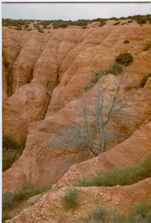
12.11-IM-AC-9755.- Aspecto de las facies fluviales proximales del Sistema de La Valduerna en las proximidades de Castrillo de La Valduerna. S. de La Valduerna. (9 y 10).
