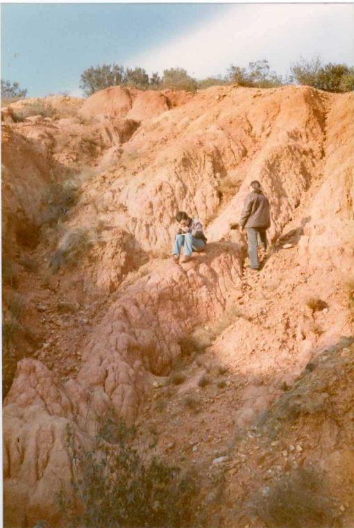
12.11-IM-AC-9758.- Aspecto de los flancos de llanura de inundación del Sistema de La Valduerna. Tramos 10 y 11 de la Serie de Herreros de Jamuz. (12-11-05). S. de La Valduerna. (9 y 10).
