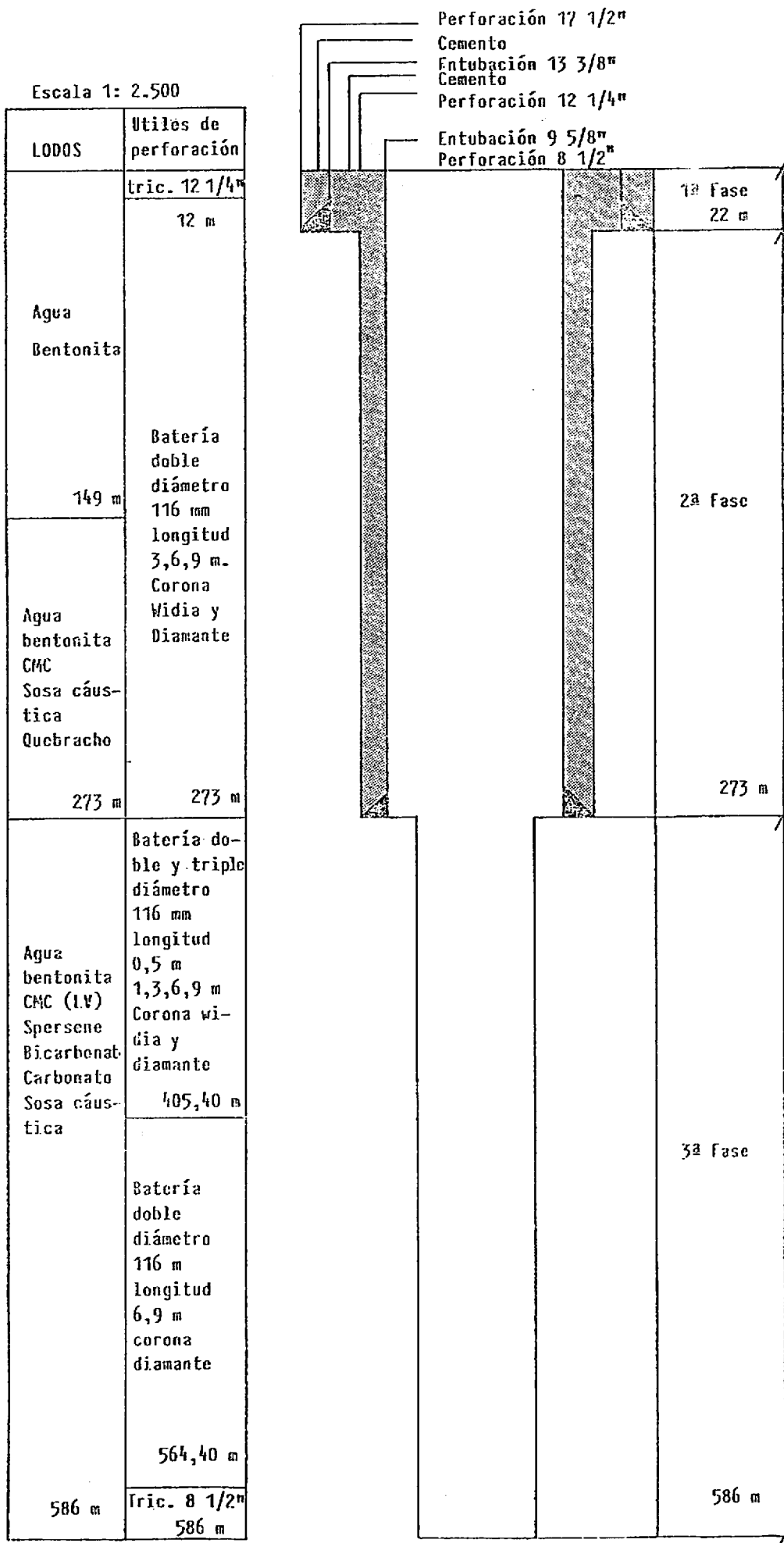
Fig. 4. Desarrollo del Sondeo Sasamón 1
