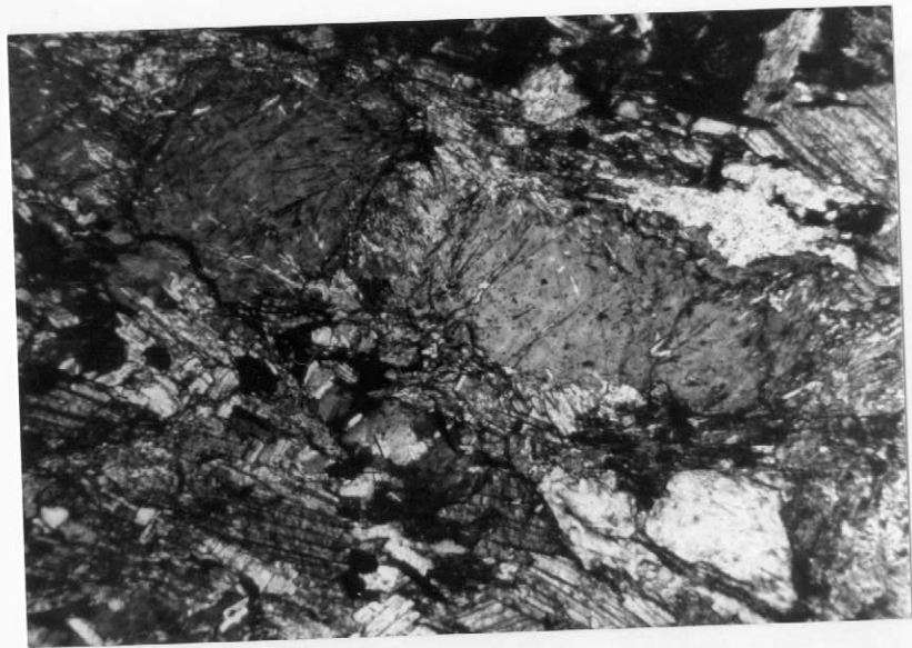
0708-IM-NB-0528 .-Fibrolita en cuarzo . LPx2 , D 78
