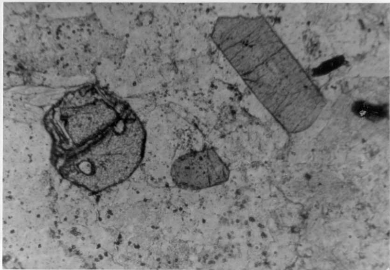
0708-IM-FR-0080.-Cristales idiomórficos de Turmalina y granate con inclusiones .LNx2,D78
