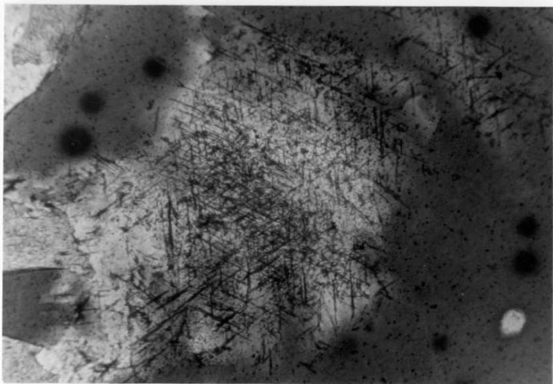
0708-IM-FR-0087.-Idem que la anterior (detalle). LNx2 ,D 78 .
