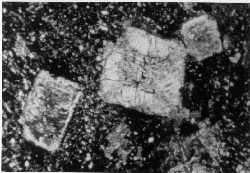
0708-IM-FR-0087 .-Microclina sustituyendo plagiocladas en Granodiorita biotitica . LPx1 .D32
