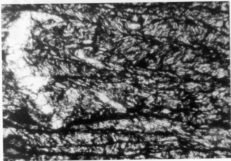
0708.-EM-FR-0092.-Esquisto crenulado . LPx2, D 78 .
