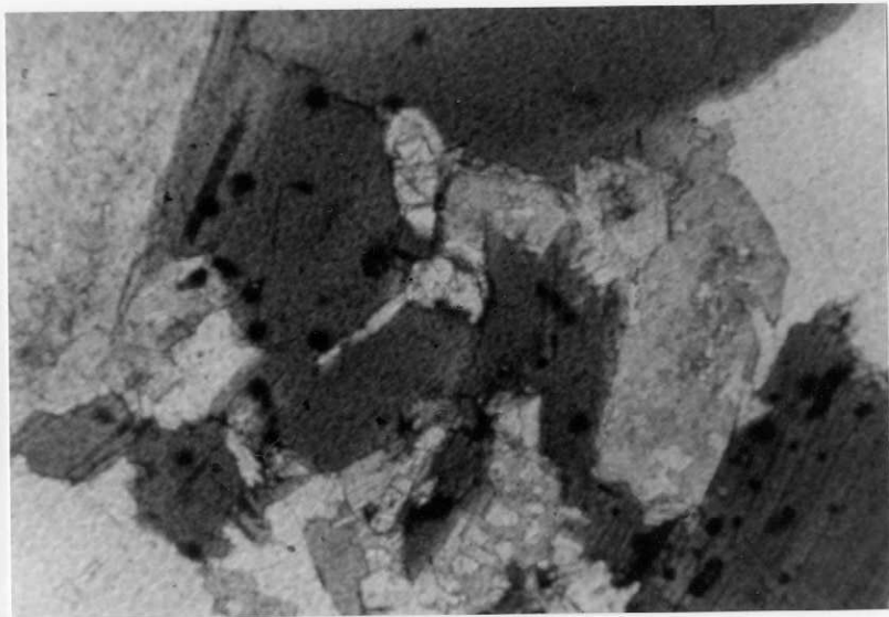
0708-IM-FR-0087.-Asociación de apatitos -biotitas en Granodiorita biotítica .LNxl , D 32.
