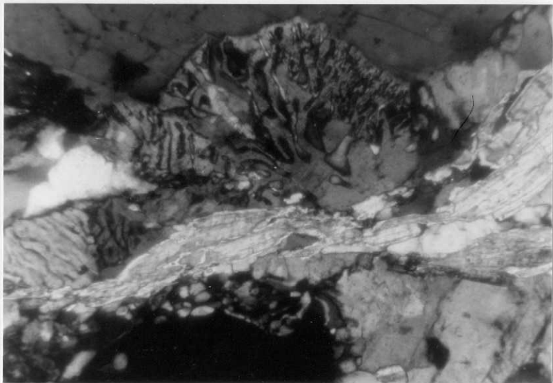
0708-IM-FR-0082 .-Mirmequitas en zonas de tectonización . LPx 3 , D 125 .
