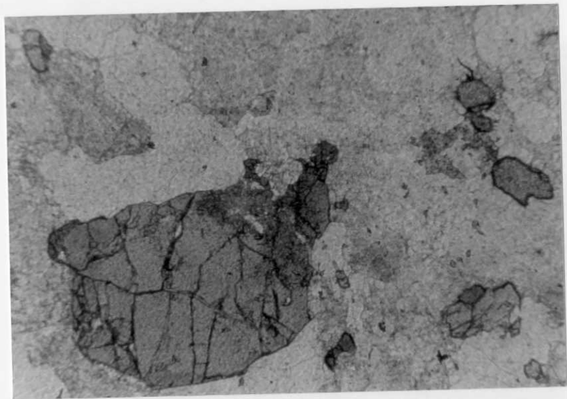
0708-IM-FR-0077.-Idem que la anterior . LNxl , D 32 .
