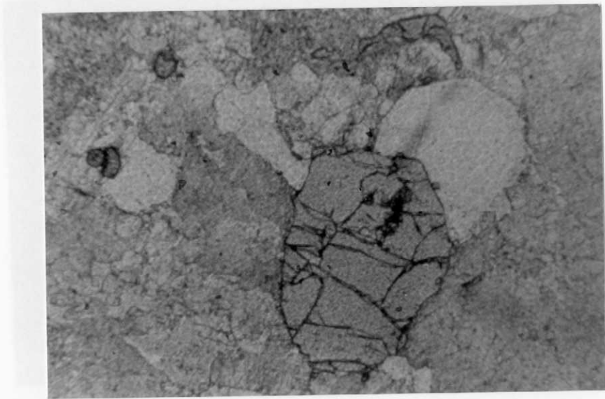
0708-IM-FR-0077.-Turmalina fracturada y granates finos en granito de dos micas . LNxl,D32
