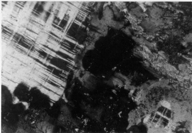
0708-IM-FR-0087.-Plagioclasa sustituida por microclina con orlas entre ambas .LPx2 , D 78
