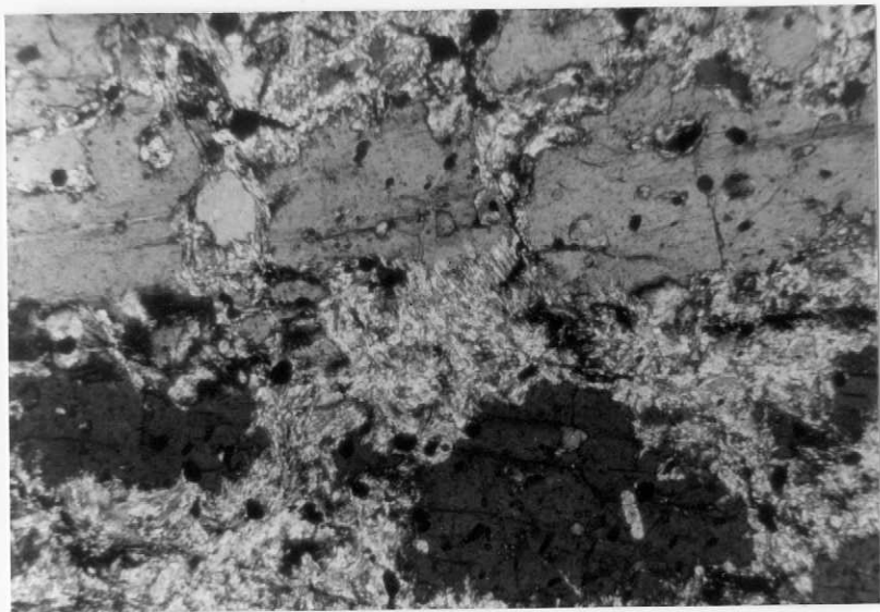
0708-IM-FR-0088.-Andalucitas relictas y moscovita -sericita. Esquisto corneanico.LPx2,D 78 .
