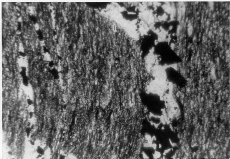
0708-IM-FR-0089.-Aspecto de lidita con filoncillos ricos en opacos .LPx2,D 78.
