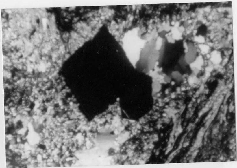
0708-IM-FR-0096.-Cristal de pirita en banda s cuarcíticas . LPx2, D 78 .
