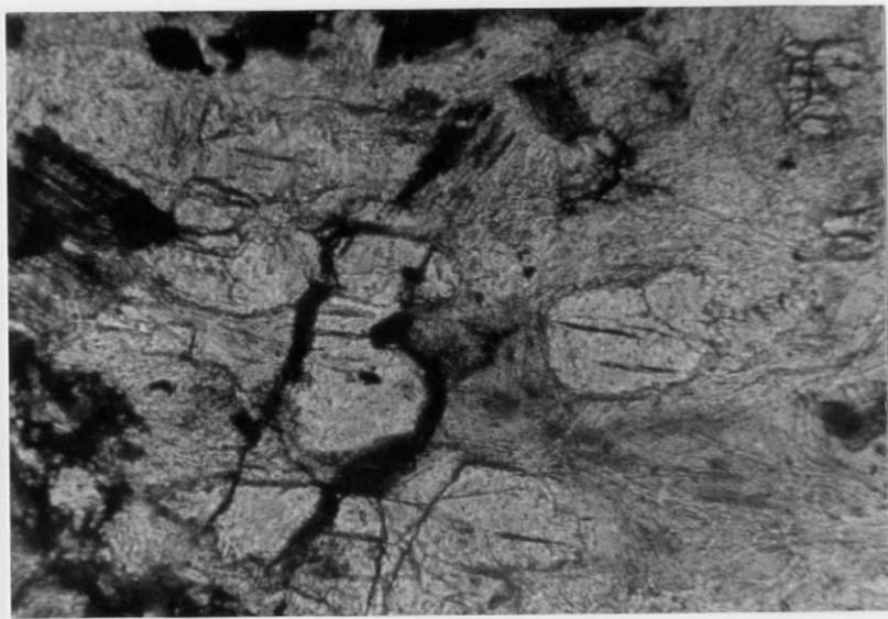
0708-IM-FR-0081 .-Andalucita relictas en moscovita fibrolítica . LNx2 ,D 78
