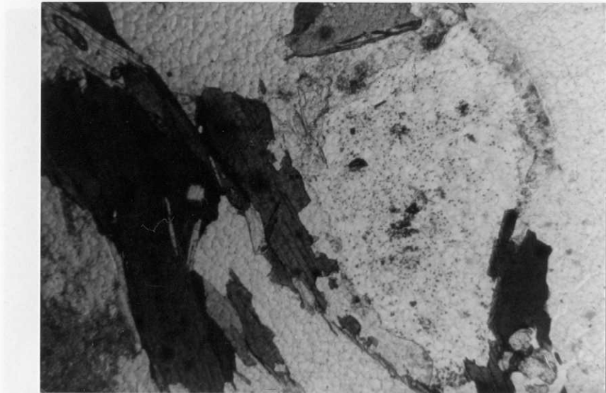
0708-IM-NB-0556 .-Biotitas orientadas en la Granodiorita Precoz .LNxl ,D32
