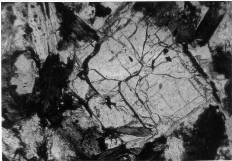
0708-IM-FR-0081.-Cristal de andalucita asociado con biotita .LNx2 ,D 78
