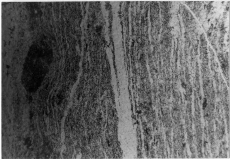
0708-IM-0512.-Aspecto bandeado de Lidita . LNx1 ,D 320
