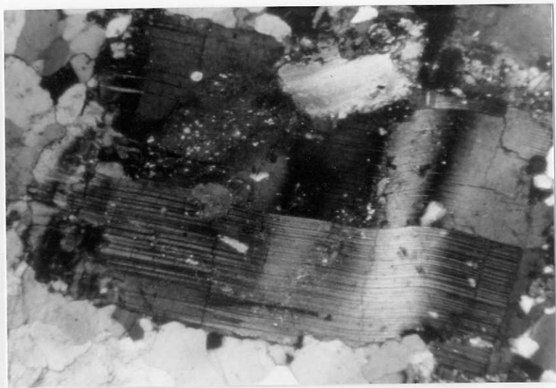
0708-IM-FR-0090.-Idem que la anterior . LPx2 ,D 78 .
