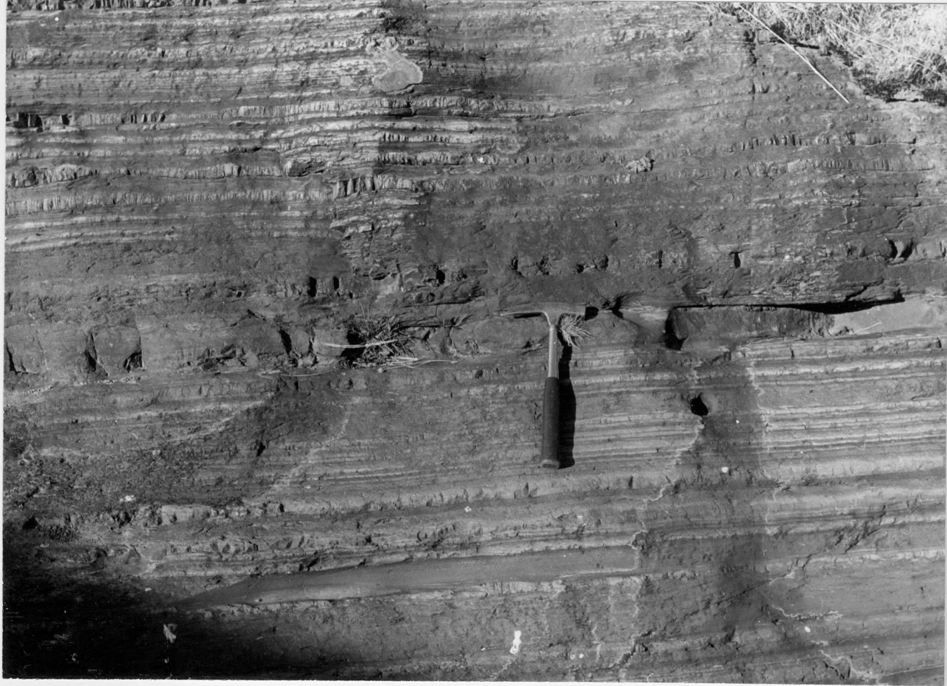
17-06-AD-MR-2213 . - Niveles de calizas ( H_{c_{24-20}}^{B-3} ) interestratificadas en las turbiditas de la Formación Vañes ( H_{cs_{22-20}}^{B3-B1} ).
