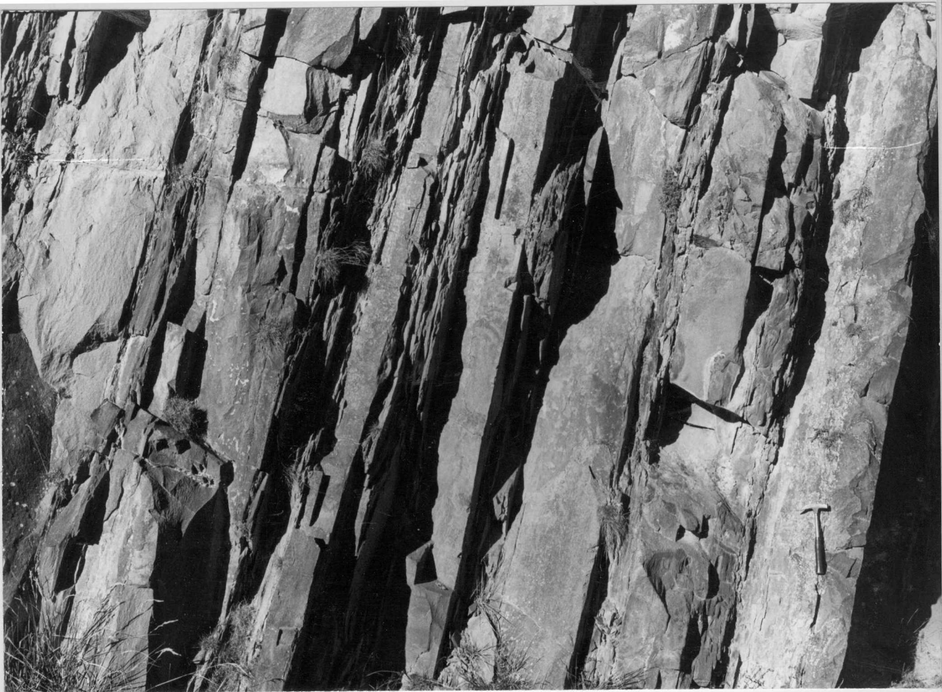
17-06-AD-MR-2204. - Grauvacas masivas de la Formación Carmen ( B-2 Hs 22-2B)
