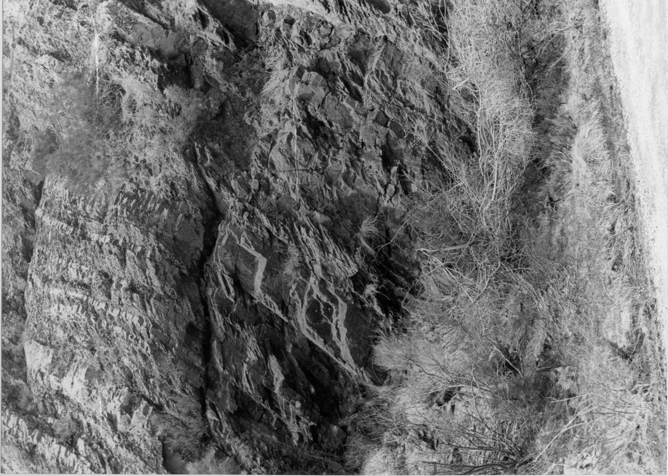
17-06-AD-MR-2209. - Turbiditas de la Formación Vañes (H 25 B3-B1 22-20 ). .
