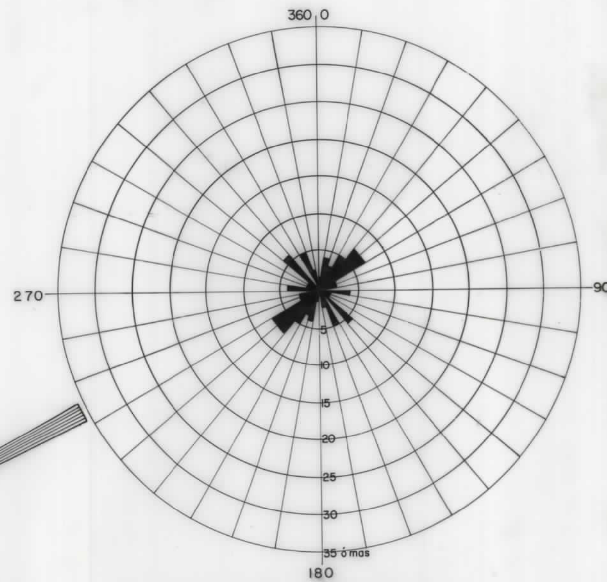
DIACLASAS MACIZO CASTROVERDE 51 DIACLASAS CONSIDERADAS SUBVERTICALES
