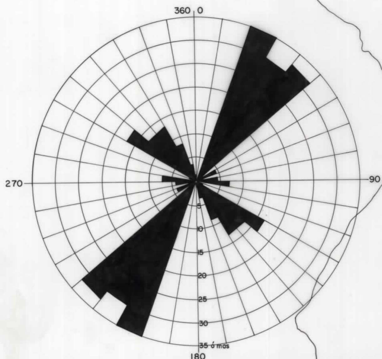
DIACLASAS MACIZO LUGO (176 DIACLASAS CONSIDERADAS SUBVERTICALES)
