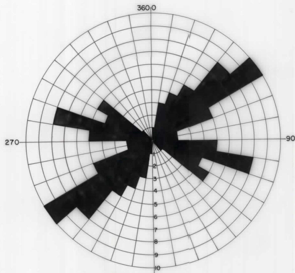
FALLAS PALEOZOICO 63 FALLAS CONSIDERADAS SUBVERTICALES
