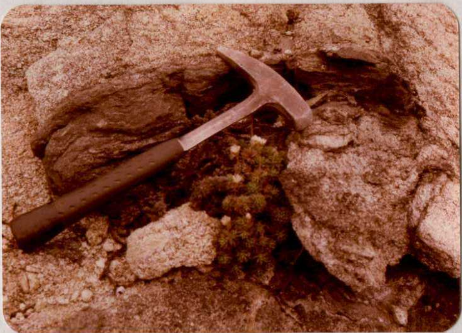
0206-IMRA -0540.- Vista de un dique de Vaughneritas cerca de Cabo Toriñana .
