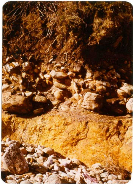
0206-IM-RA-0526.-Depositos basales de la rasa en la playa de Charente(Ensenada de Merejo).
