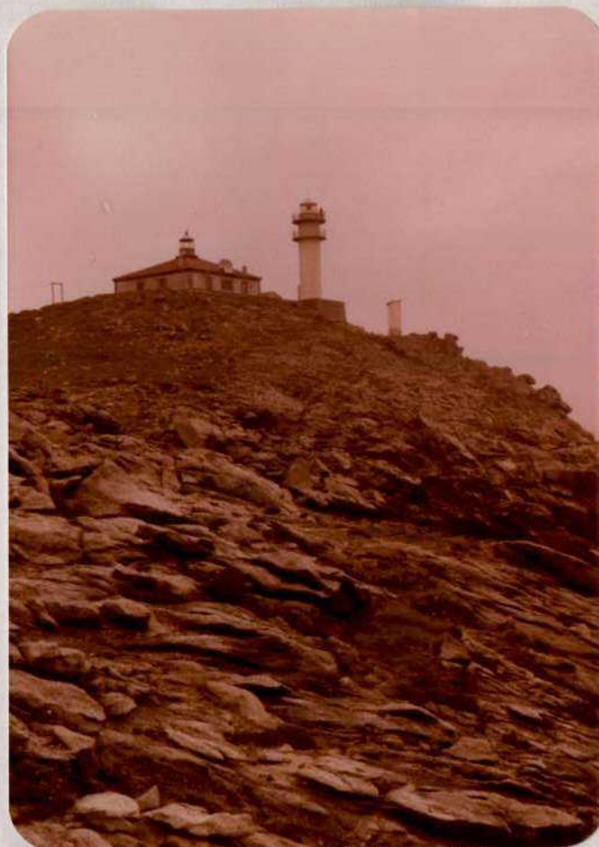
0206-IM-RA-0542 .-Aspecto topográfico del granitoide migmatítico homogéneo en Cabo Toriñana .
