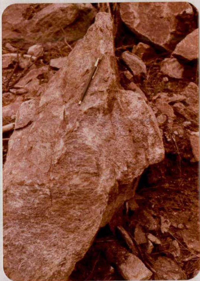
0206-IM-RA-0536 .-Aspecto inhomogeneo del granitoide migmatítico .
