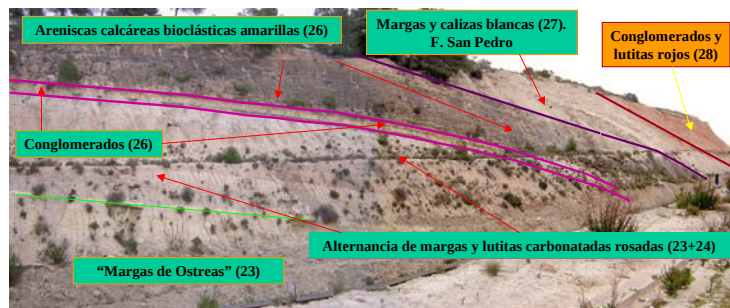
Foto 45.- La serie del Puerto de San Pedro a lo largo de l ferrocarril Murcia-Cartagena. Posiblemente sea uno de los afloramientos de mejor calidad para observar el registro sedimentario del transito Mioceno-Plioceno en los sectores NE de la Cuenca del Campo de Cartagena.
