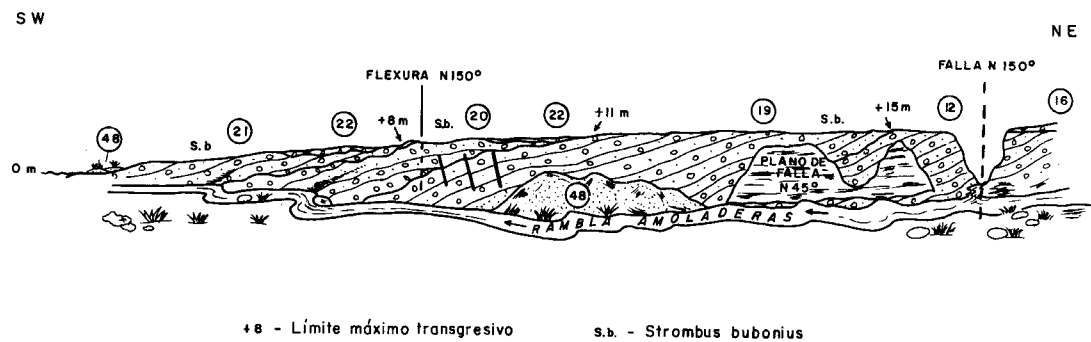
Fig. 2 .- Disposición de los materiales cuaternarios en rambla Amoladeras
