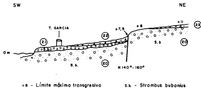
Fig. 3 .- Disposición de los materiales cuaternarios en relación con la neo-tectónica. Alrededores de Torre Garcia.
