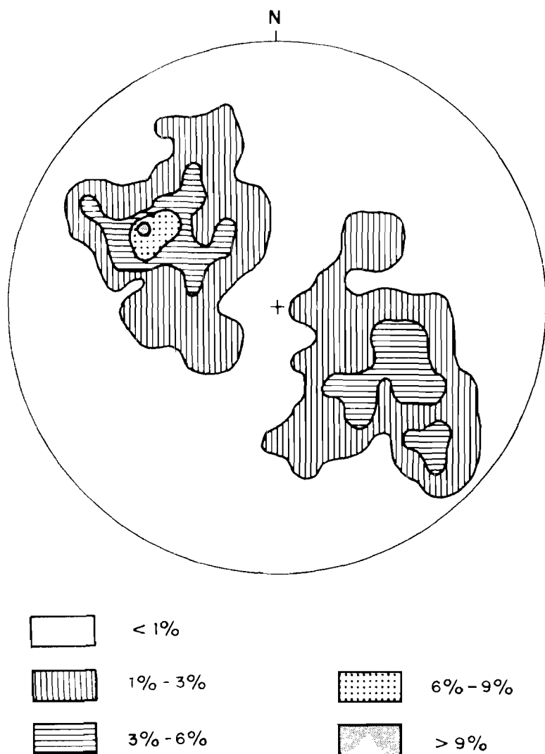
Figura núm. 2.—Proyección de 132 polos de la lineación de intersección L_1 . Falsilla de SCHMIDT (hemisferio inferior).
