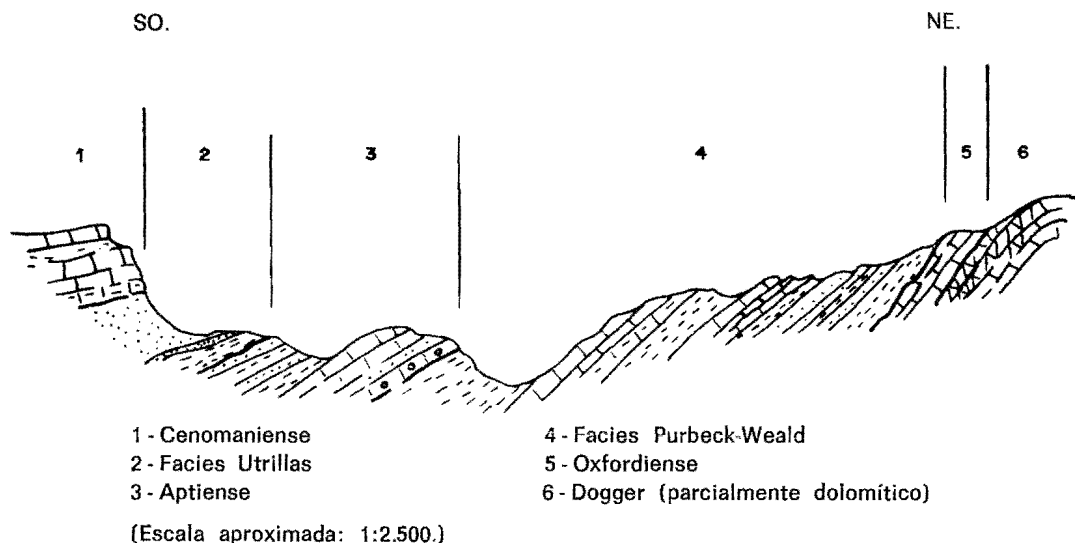
Figura 6 bis.—Corte esquemático en la terminación periclinal del anticlinal jurásico de Valdelacasa, al NE. de Algarra.
