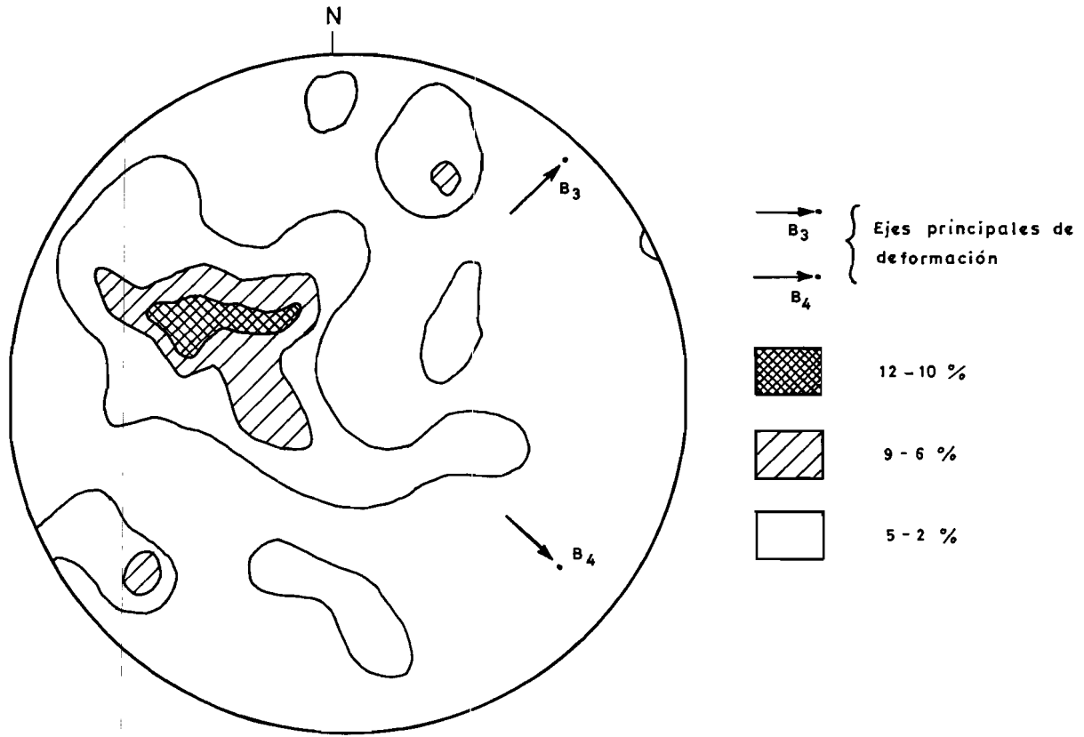
Fig. 3.— Proyección Estereográfica de esquistosidades (H. Inferior) (50 datos).
