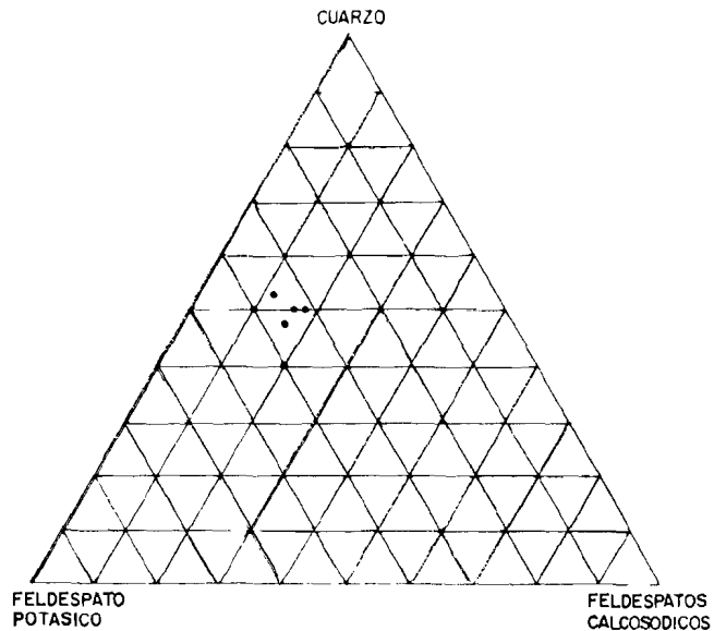
Figura 14.—Composición mineralógica de las arenas de la Unidad de Arévalo.
