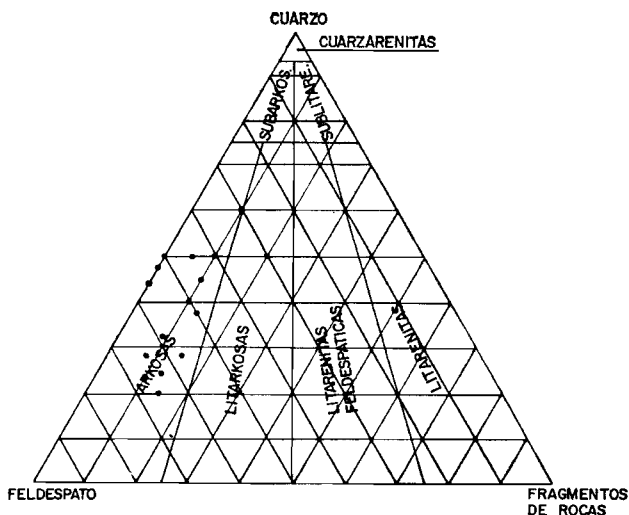
Figura 11.—Composición mineralógica de las arenas de la Unidad Peromingo.
