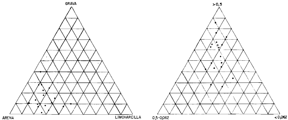
Figura 12.—Composición granulométrica de las arenas de la Unidad de Peromíngos.
