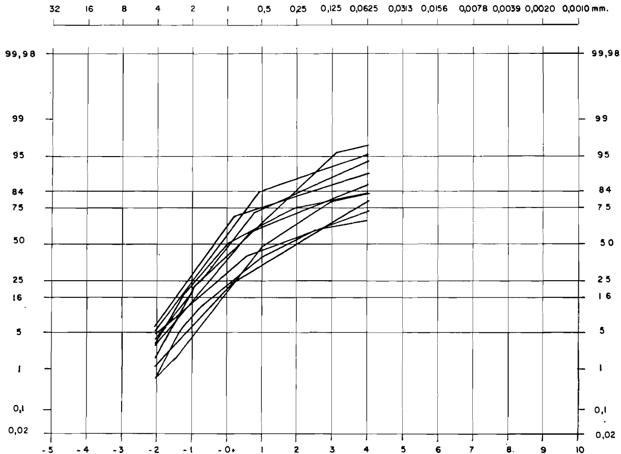
Figura 4.—Curvas granulométricas de las arenas de las Unidades de Pozanco (16-20) y Vallehernando (15-20).
