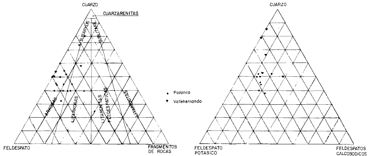
Figura 2.—Composición mineralógica de las arenas de las Unidades de Pozanco (Hoja 16-20) y Vallehernando (15-20).
