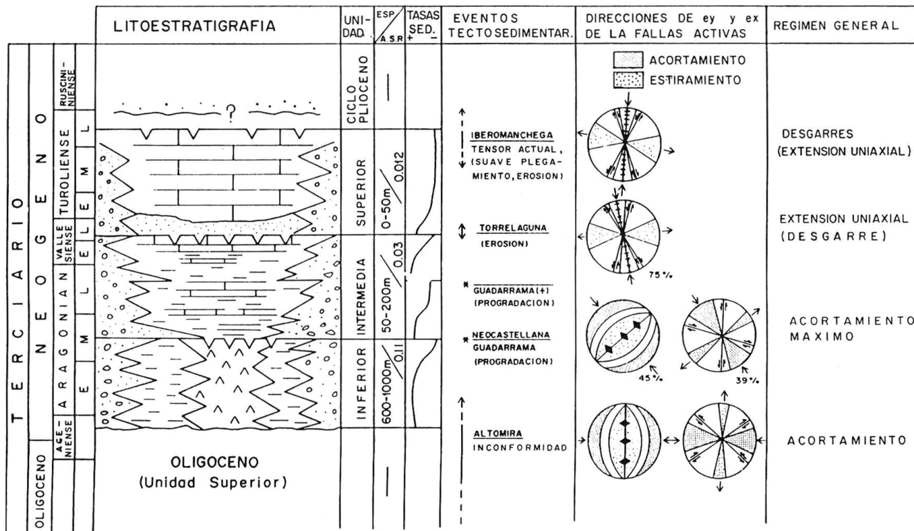
Figura 5.2. Cuadro de correlación entre unidades tectosedimentarias y campos de esfuerzo en la cuenca de Madrid durante el Neogeno (según Calvo et Al. 1991).
