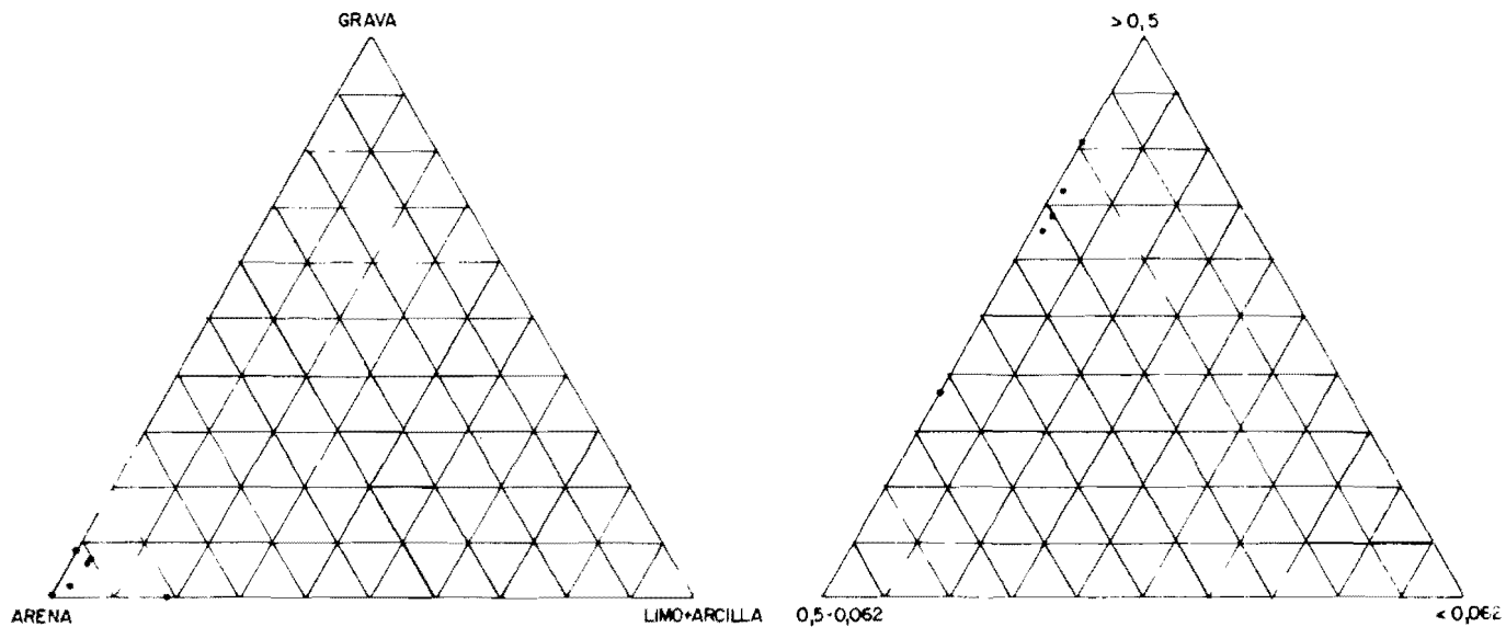
Figura 13.—Composición granulométrica de las arenas de la Unidad de Arévalo.
