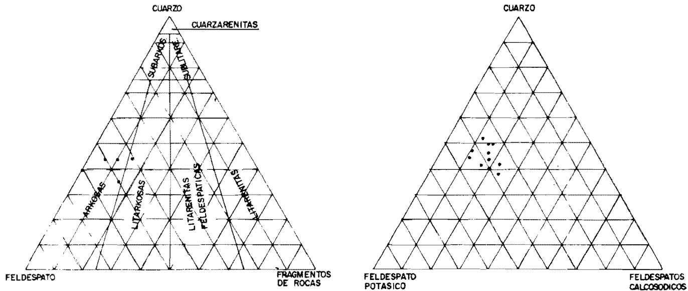
Figura 9.—Composición mineralógica de las arenas fluviales (terrazas).
