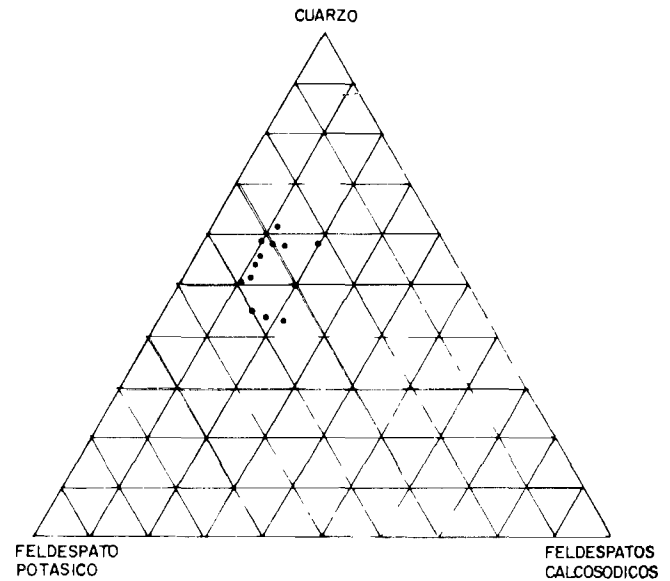
Figura 15.—Composición mineralógica de las arenas eólicas.
