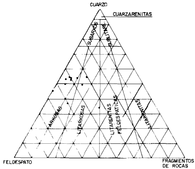
Figura 15.—Composición mineralógica de las arenas eólicas.
