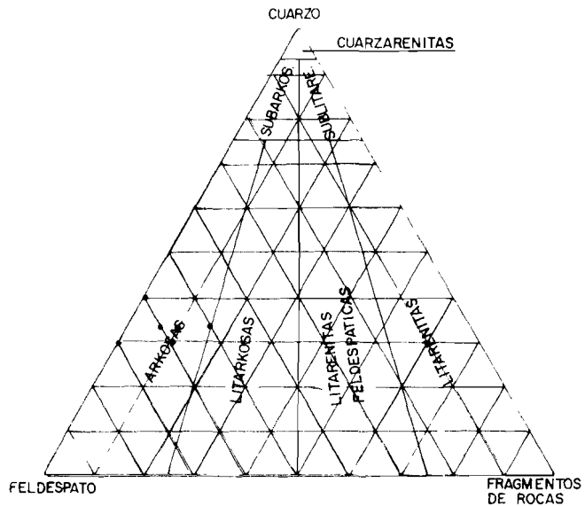
Figura 12.—Composición mineralógica de las arenas de la Unidad de Arévalo.
