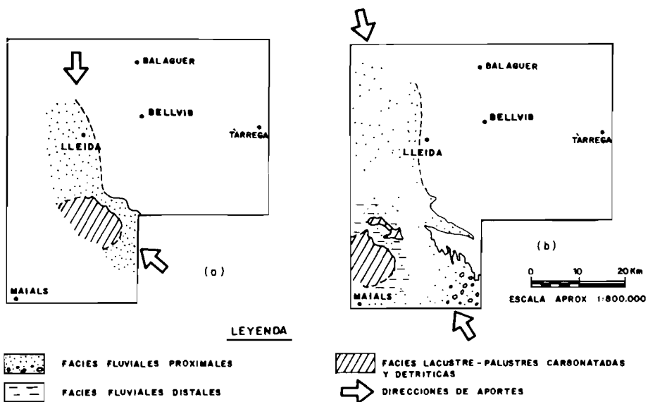
Fig. 2. Esquemas de distribución de facies de las unidades genético-sedimentarias de Castellidans (a) y Alfés (b)
