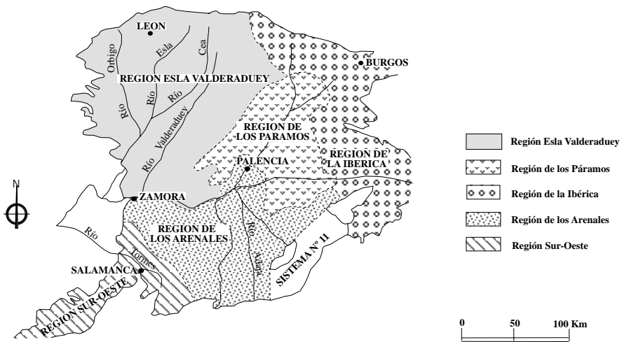
Fig. 6.- Distribución de los Sistemas Acuíferos en la Cuenca del Duero. (Tomada de Navarro et.al. 1989).
