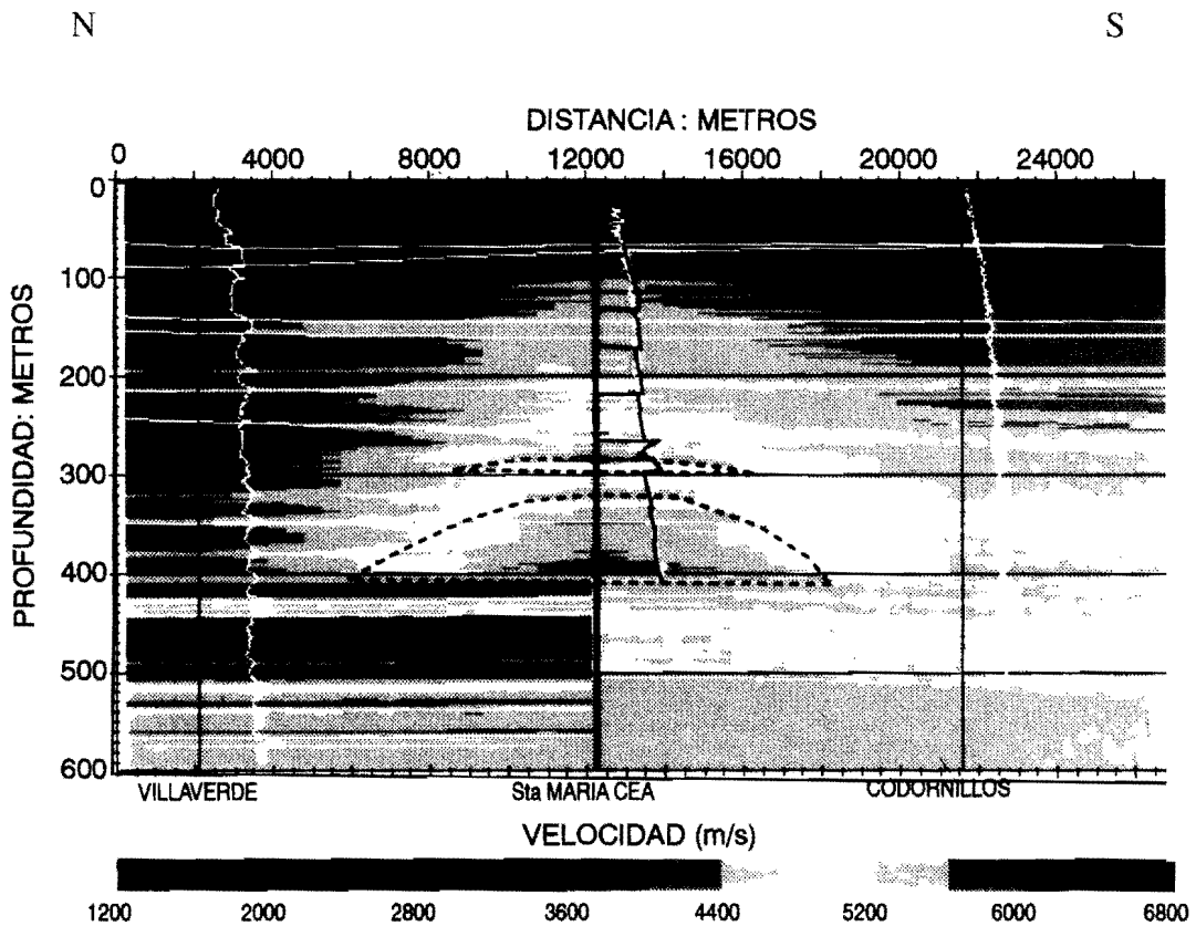
Fig 2.7.- Correlación de diagrfias sónicas o de velocidad, corte CVEL-5
