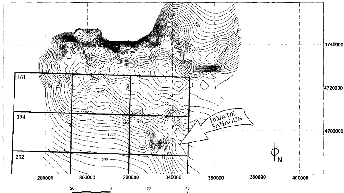
Fig. 3.6.- Mapa de Isobatas (datum 900 m. s. m.) del techo de las calizas del Crétacico Superior-base del Terciario. Sector NO. de la Cuenca del Duero y referencia a las Hojas estudiadas; intervalo de contornos 100 m. Tomada de Redondo et. al. (1995).
