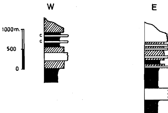
Figura 3.—Columnas estratigráficas esquemáticas de los niveles basales de la Formación Agüeira a ambos flancos del sinclinal de Ibias. En blanco, niveles con areniscas dominantes; rayado, alternancia de siltitas, pizarras y areniscas; negro, pizarras; c, cuarcitas. Los niveles de areniscas corresponden a turbiditas A o B y los niveles rayados a turbiditas C, predominantemente.
