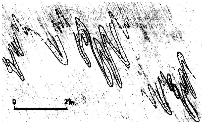
Figura 4.—Pliegues isoclinales correspondientes a la primera fase de deformación en niveles de areniscas de la Formación Agüeira (cerca de Puente Boadil).
