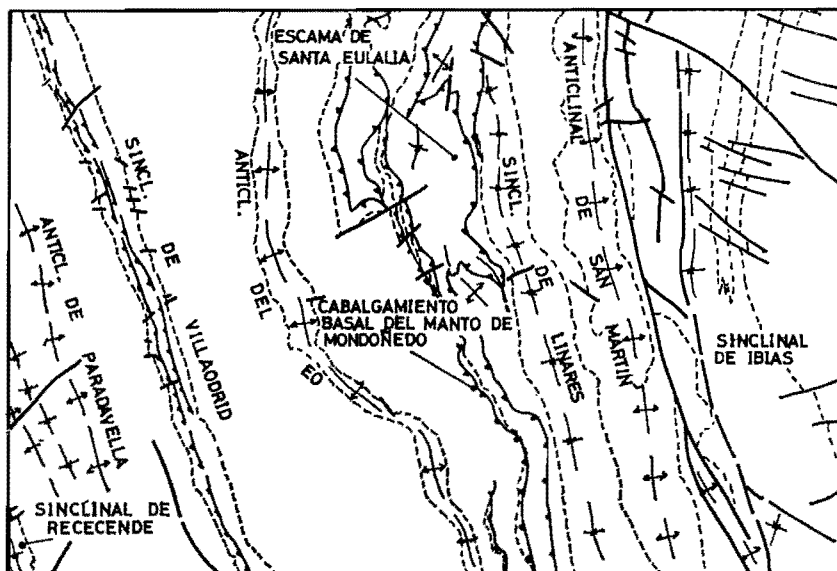
Figura 2.—Esquema de situación de las principales estructuras mencionadas en el texto.
