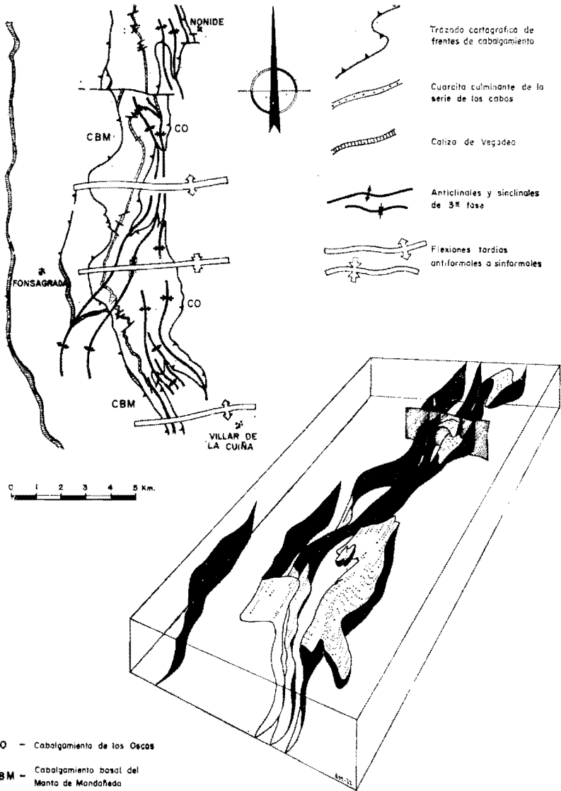
Figura 5.—Replegamiento de la superficie de cabalgamiento de la escama de Santa Eulalia de Oscos, al E. de Fonsagrada, según MARCOS (1973).
