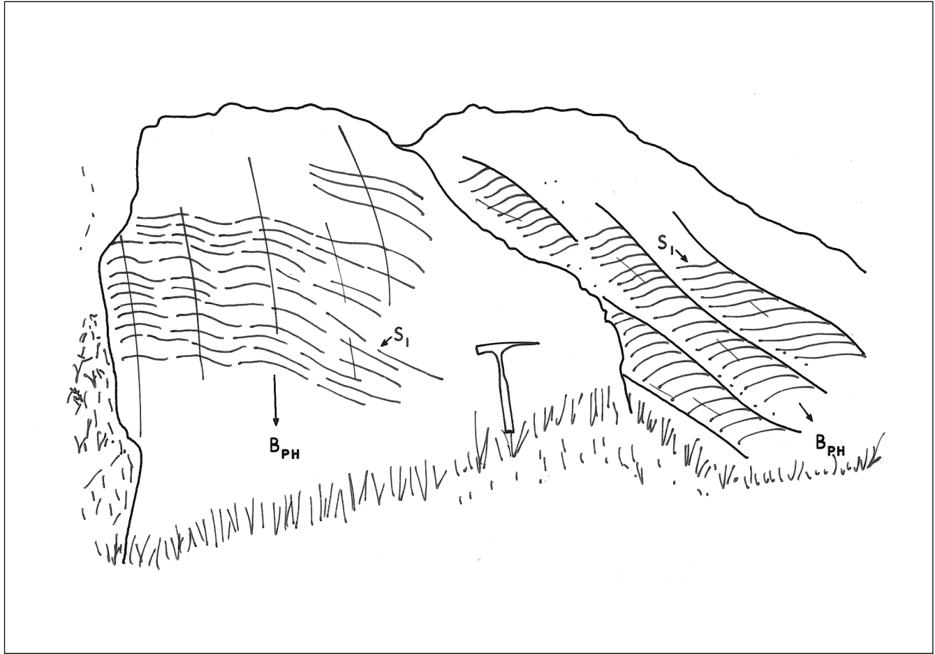
Figura 3.2. Charnelas prehercínicas suavemente onduladas en el flanco de un pliegue de 1.ª fase hercínica con S_1 según la dirección del mismo.
