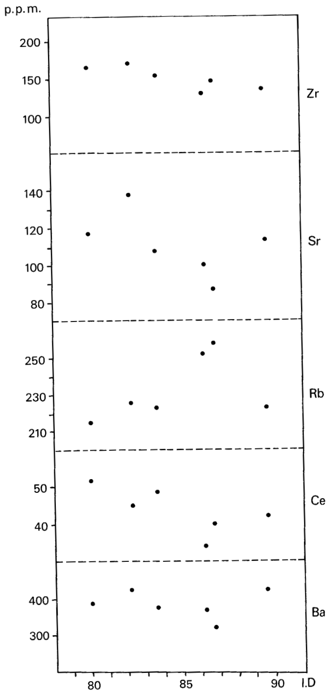
FIG. 11 Representacion de algunos de los elementos menores frente al índice de diferenciacion.
