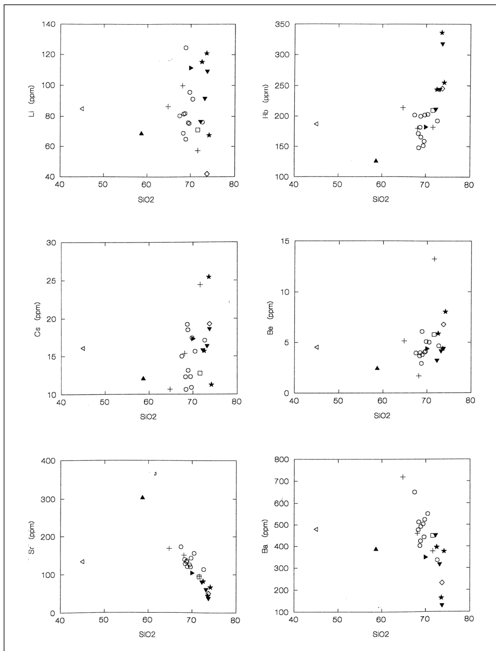
Figura 7. Diagramas de HARKER: elementos traza de muestras de la hoja de Navaluenga.
