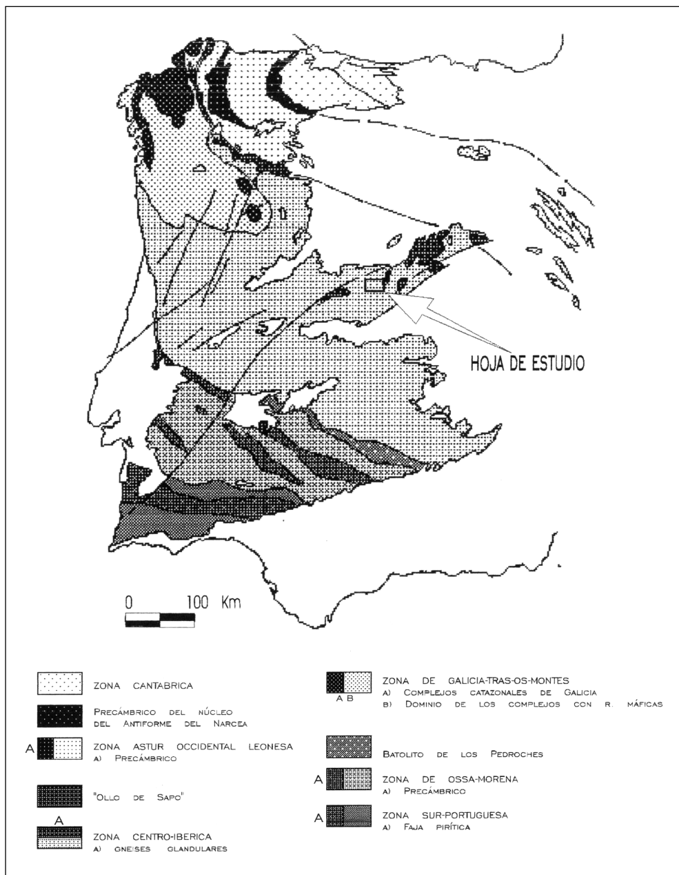
Figura 1. División en zonas del Macizo Ibérico, modificado de JULVERT et al. (1972), según MARTÍNEZ CATALÁN (1981). Situación de la Hoja de Navaluenga.
