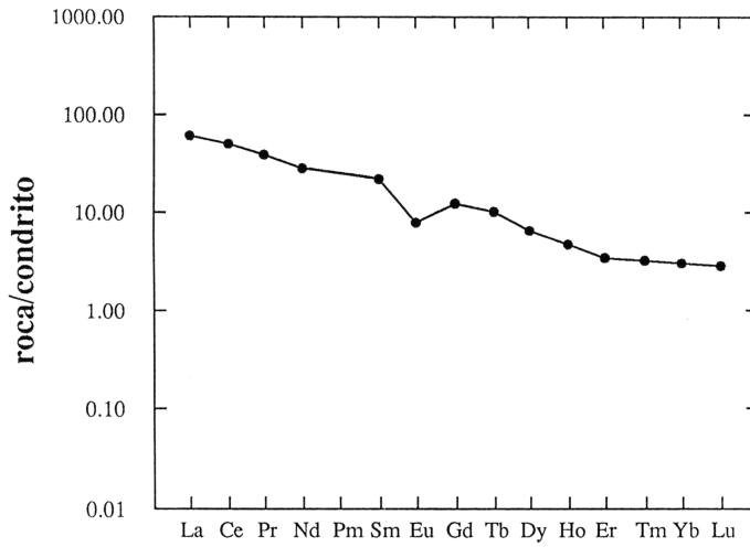
Figura 17. Espectro normalizado de tierras raras del leucogranito aplítico tabular (20).
