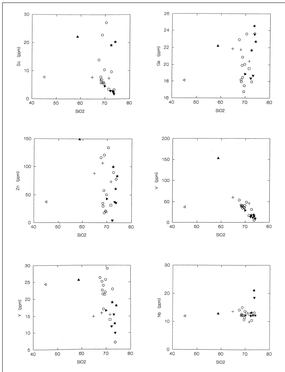
Figura 8. Diagramas de HARKER: elementos traza de muestras de la hoja de Navaluenga.
