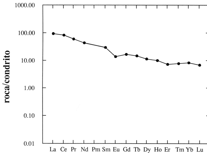
Figura 18. Espectro normalizado de tierras raras de pórfidos (1).
