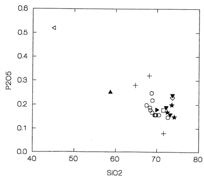
Figura 6. Diagramas de HARKER: elementos mayores de muestras de la hoja de Navalunga.
