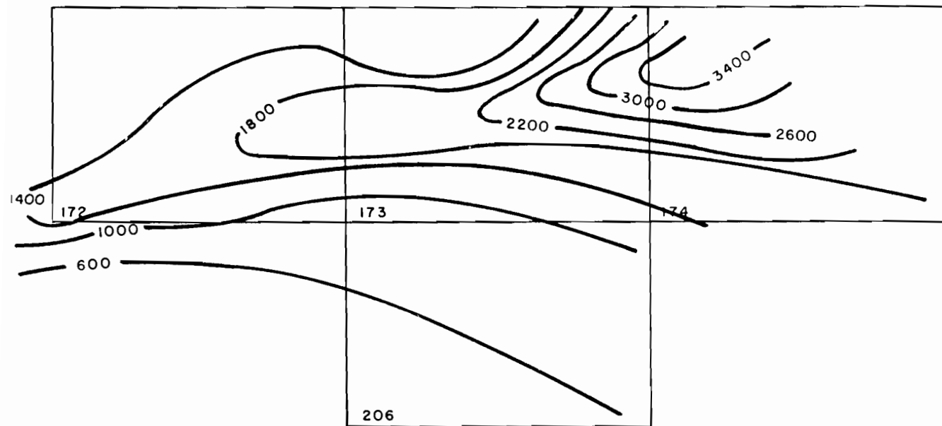
Fig. 6.— Mapa de isopacas de las unidades detríticas de la 3ª UTS (U. Rocaforte+ U. de Sangüesa+ U. de Leoz + U. de Allo+ U. de Larraga).
