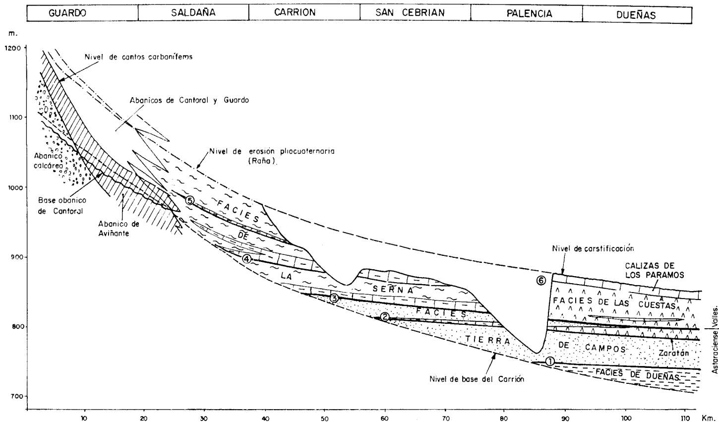
Figura 1.—Esquema estratigráfico.
